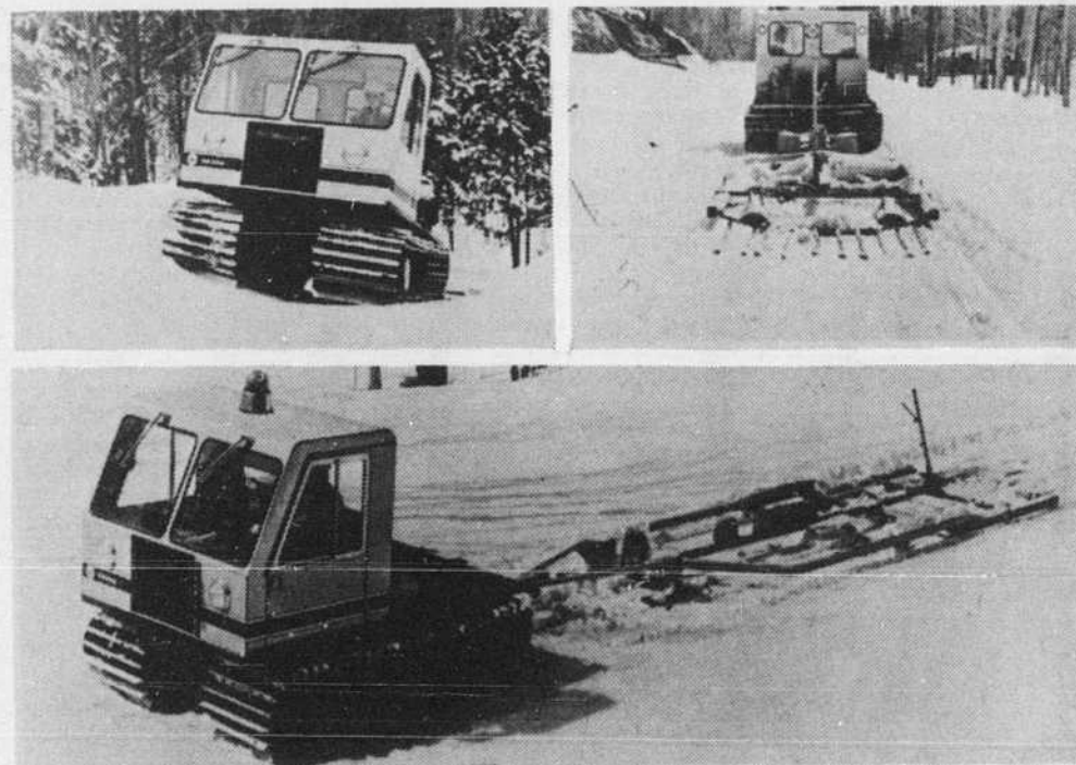
Voici le dernier-né de la firme québécoise Bombardier, le Skidozer SV-200 qui est le plus petit modèle de la série des trois d'après la division industrielle de la compagnie pour entretenir les pentes de ski et les chantiers. C'est la version économique du Skidozer 250 qui s'était mérité des prix d'esthétique industrielle en janvier dernier au Congrès national de l'entretien organisé aux États-Unis.
