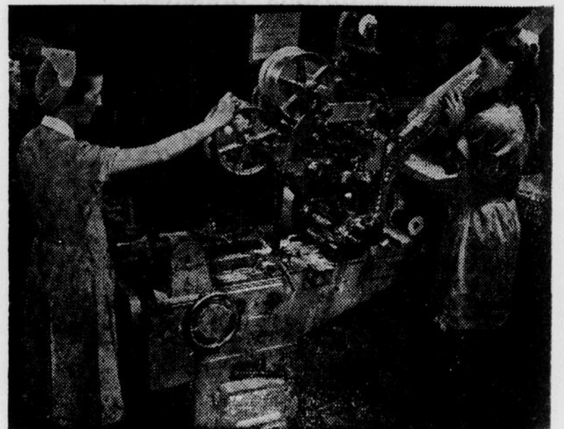
Cet appareil enveloppe dans la pellicule cellulosique "Cellophane" quelque 200 paquets de cigarettes à la minute. Le Canada suffit à presque 98 pour cent de sa consommation de tabac, alors qu'en 1930, il en importait près de 60 pour cent.
