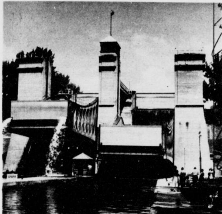
LES DEUX BASSINS en mouvement simultané. Ils se font équilibre. Quand l'un monte, l'autre descend. Pour rendre plus léger celui qui monte, on lui laisse échapper un peu d'eau, comme on peut le constater.
