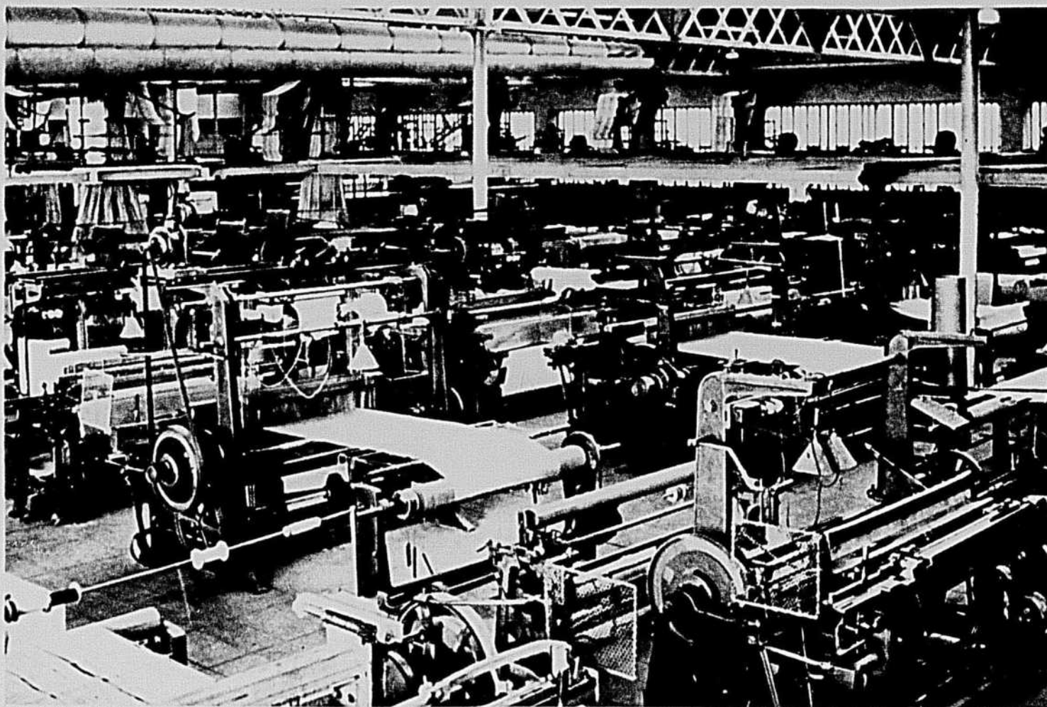
L'école de tissage de Lyon: Une salle de métiers pour tissus unis.
