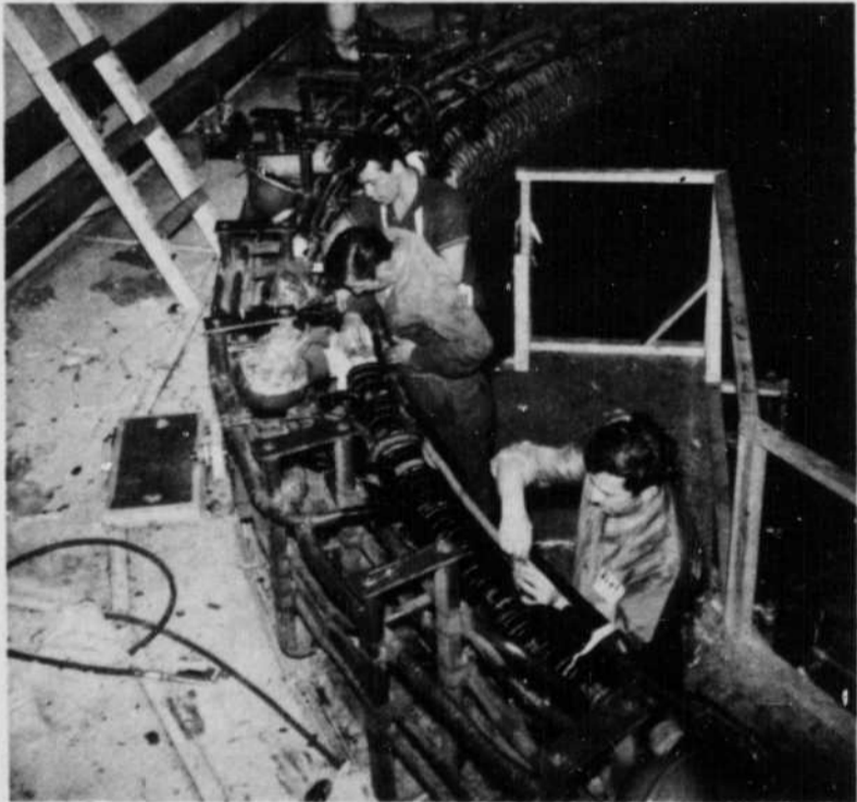
NETTOYER - REPARER — Trois employés de la centrale de Chute-des-Passes refont les joints sur les bobinages d'un stator que l'on vient de mettre à jour après avoir sorti le rotor. Ce sont MM. J.-E. Gauthier, J.-P. Tremblay et R. Asselin.
