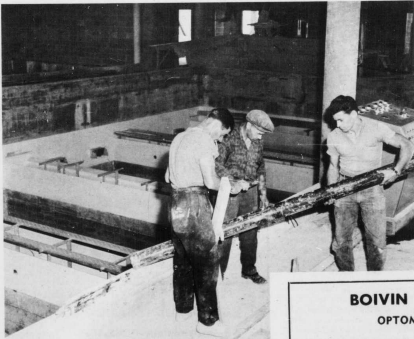
LES BASSINS sont prêts à recevoir le sable des lits filtrants. Les ouvriers s'affairent à la mise au point de la machinerie qui fera du filtre de Jonquière, une usine où l'automatisme sera maître.
