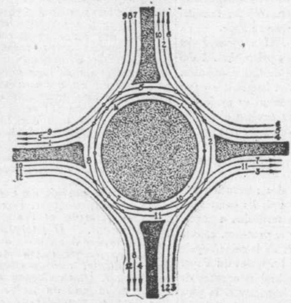
Diagramme des circuits d'un Rond-Point
