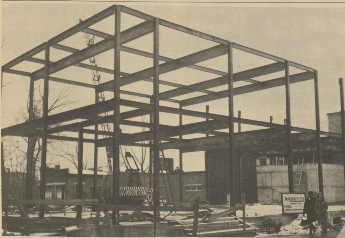
La charpente en acier du futur édifice abritant les locaux de la Caisse populaire de Saint-Jean sera parachéevée d'ici une journée ou deux, comme on peut le constater sur cette photo. Cet édifice commercial est érigé par la firme Eloi Gagnon, de Saint-Jean.
