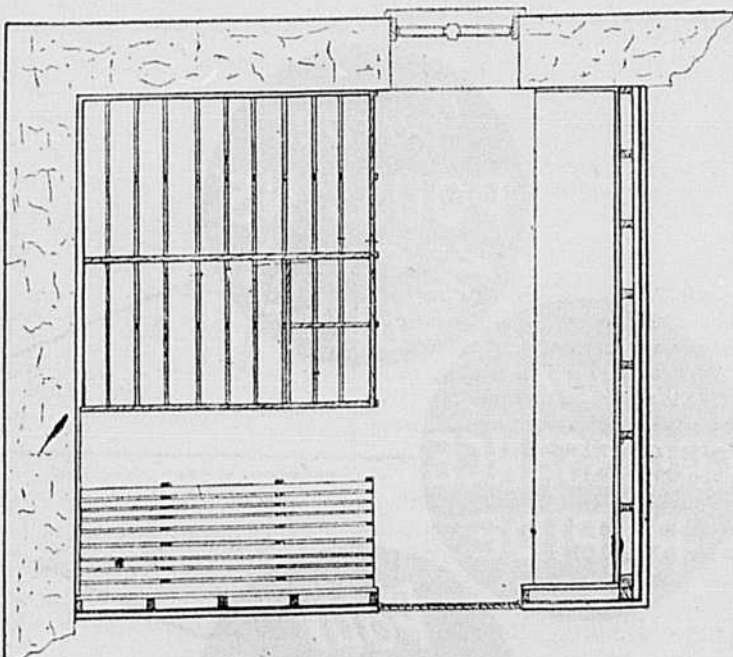
Caveau à légumes. Plan de plancher.
