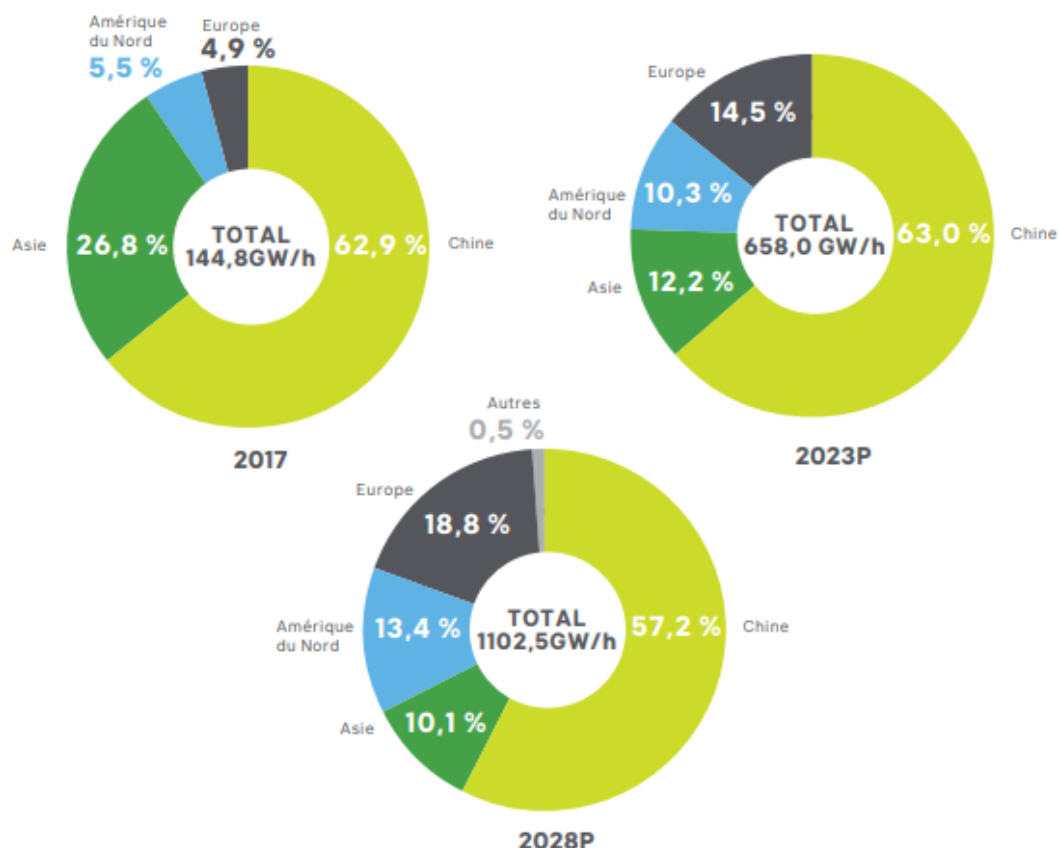
Figure 11. Capacités actuelle et annoncée de production de batteries lithium-ion dans les méga-usines, septembre 2018
