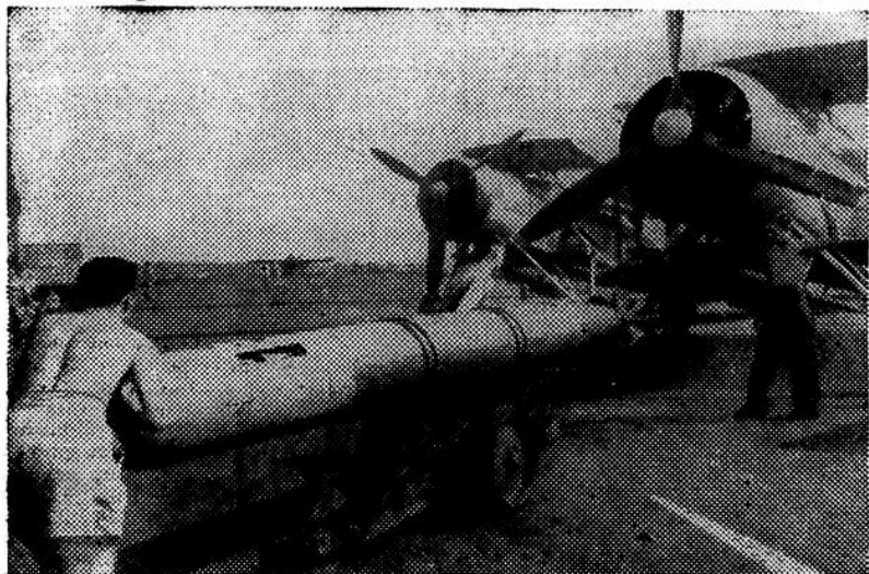
Une torpille rejoint son attache sous le fuselage d'un avion lance-torpille Swordfish, de la Marine Royale et de la RAF. La photo fut prise sur le point d'envol d'un navire porte-avion britannique.
