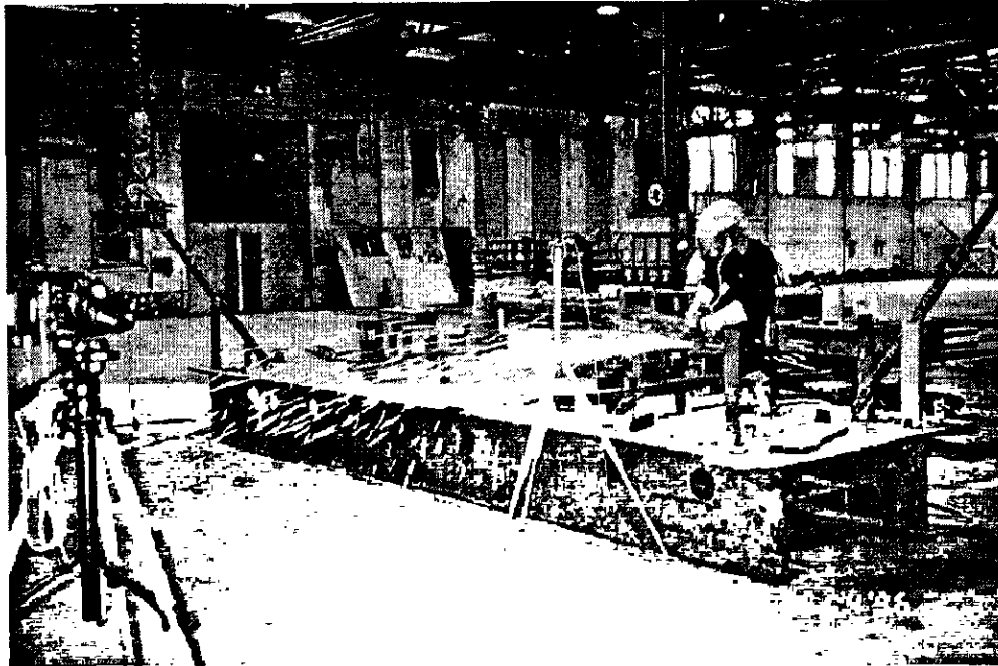
Figure 4.3 Meulage sur acier dur en position basse
