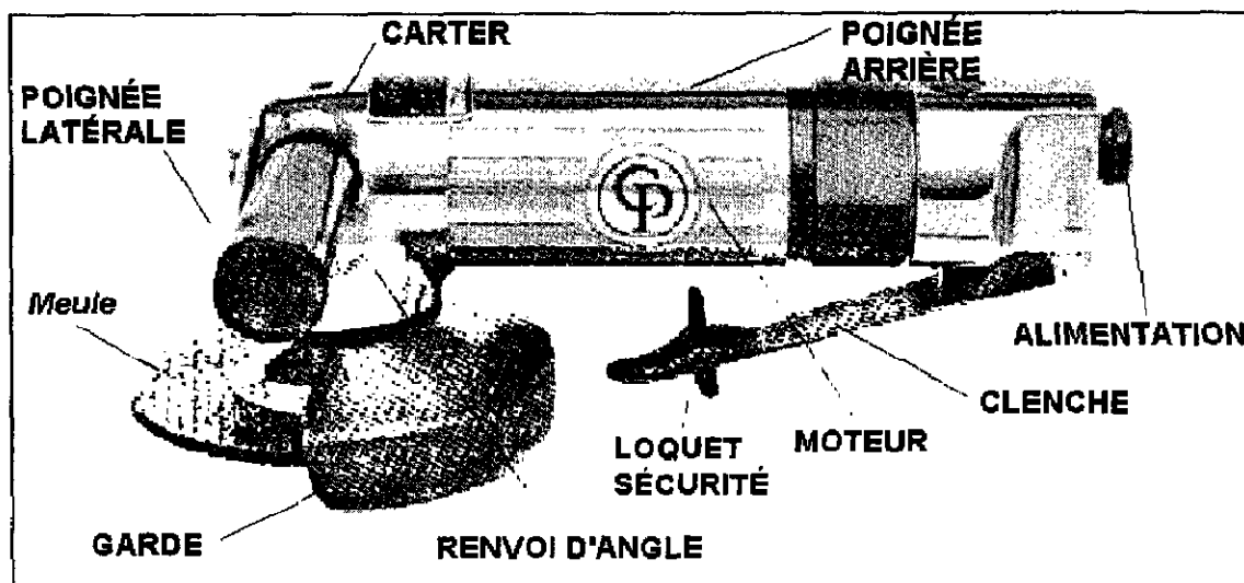
Figure 2-5 Description des principaux systèmes d'une meuleuse à angle.
