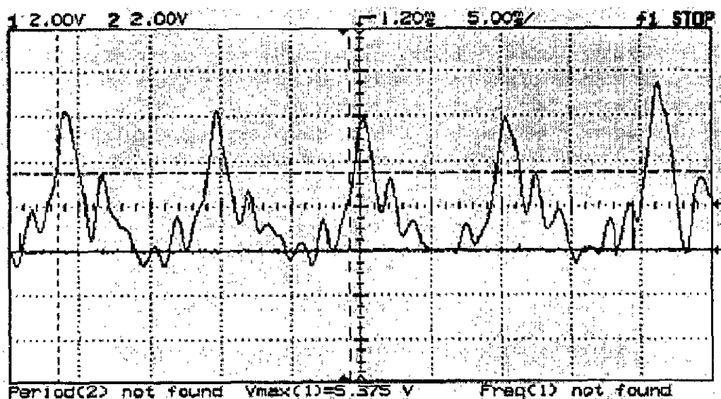
Force de coupe pour un taux d'engagement de 88 %
