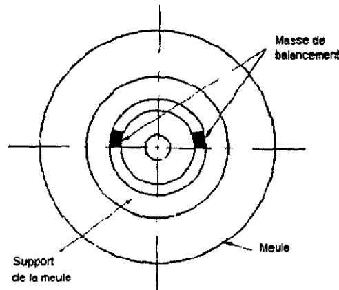
Figure 2-4 Balancement d'une meule
