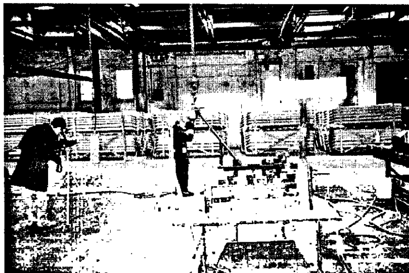
Figure 4.6 Meulage sur acier mou en position haute et enregistrement vidéo des mouvements et positions de l'opérateur.
