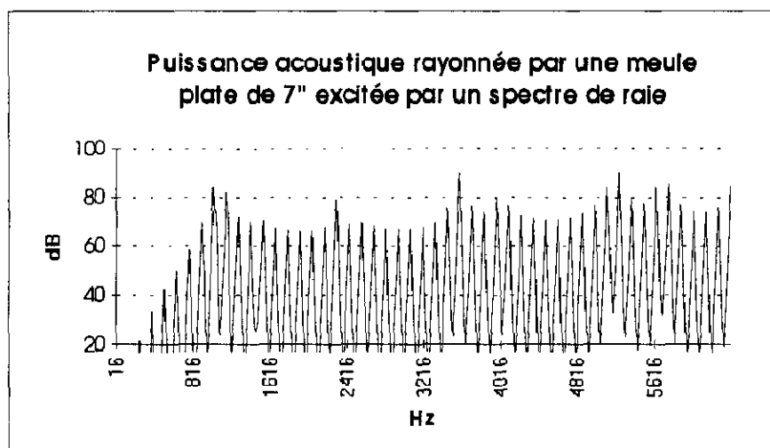
Spectre de puissance acoustique calculé
