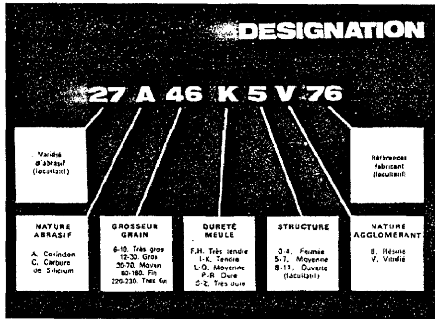
Figure 2-2 : Désignation des meules [Source: TOBELEM, W., (1988)]
