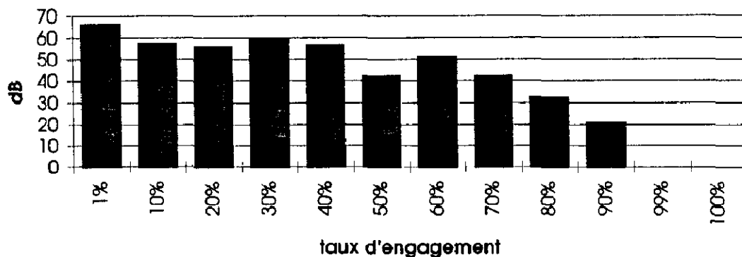
Augmentation du bruit des meules plates de 7" en fonction du taux d'engagement
