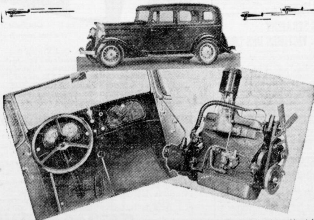
Les deux principales caractéristiques de la nouvelle six-cylindres Essex sont le prix raisonnable et l'application pour la première fois à l'automobile de certaines techniques de l'aviation. Ce fait a valu à la nouvelle voiture d'être baptisée "Terraplane". Voici, en haut, le Terraplane sedan; en bas, à gauche, une vue intérieure du tablier avant; à droite, le moteur à haute compression.
