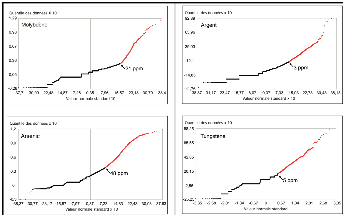
FIGURE 10 - Diagrammes quantile-quantile montrant les seuils anomaux pour le molybdène, l'argent, l'arsenic et le tungstène. Les échantillons sélectionnés sont en rouge sur la courbe.
