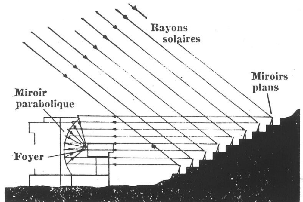
Le principe de captation de l'énergie solaire.
