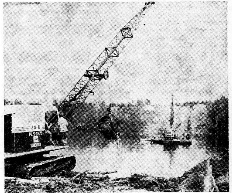
Un drag-line est à l'oeuvre sur la rive de la rivière Ground Hog, cependant que d'une barge l'on perce des trous de 6 pouces de diamètre, tous les 5 pieds, dans le lit de la rivière.
