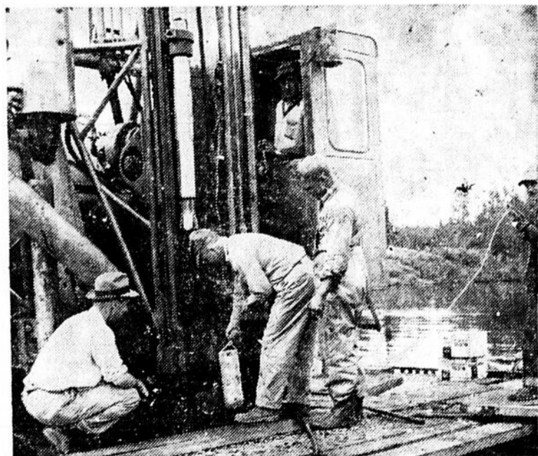
M. W.T. Copping (à g. président de l'Ontario Rock Drillers, regarde M. Lloyd Raney, spécialiste des explosifs à la Du Pont of Canada, placer une cartouche de 15 lb. dans un trou.
