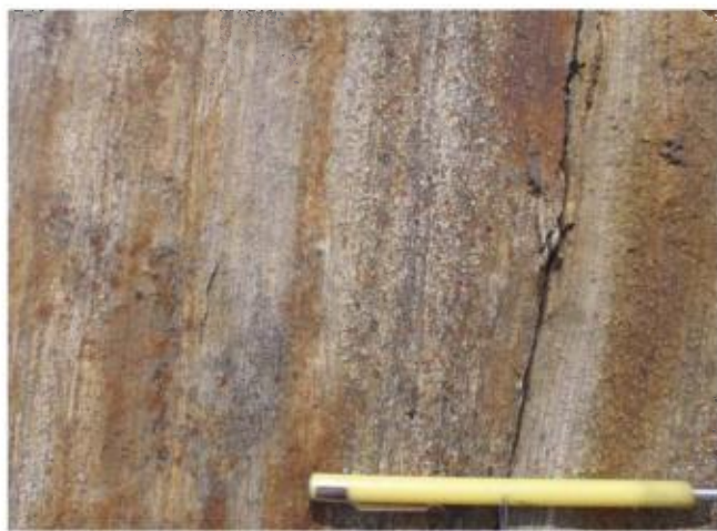
PHOTO 3 - Tuf de composition felsique à intermédiaire avec des niveaux riches en cristaux de plagioclase. Secteur avec zones rouillées de la Ceinture de Tunulic (ApPtun1).
