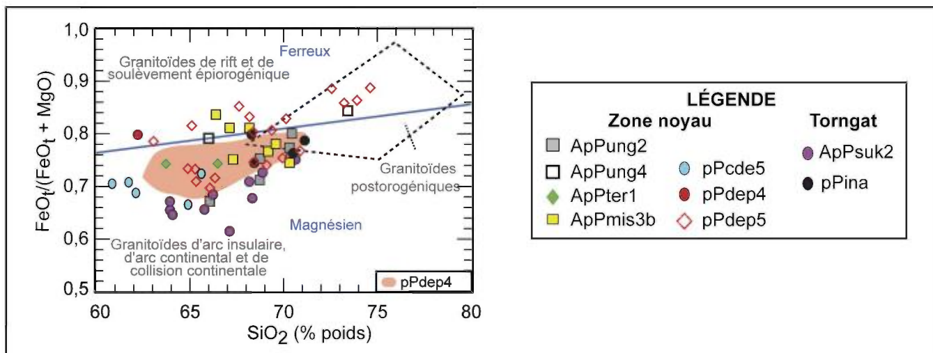
FIGURE 11 - Diagramme discriminant de Maniar et Picoli (1989) pour les roches felsiques à intermédiaires de la région
