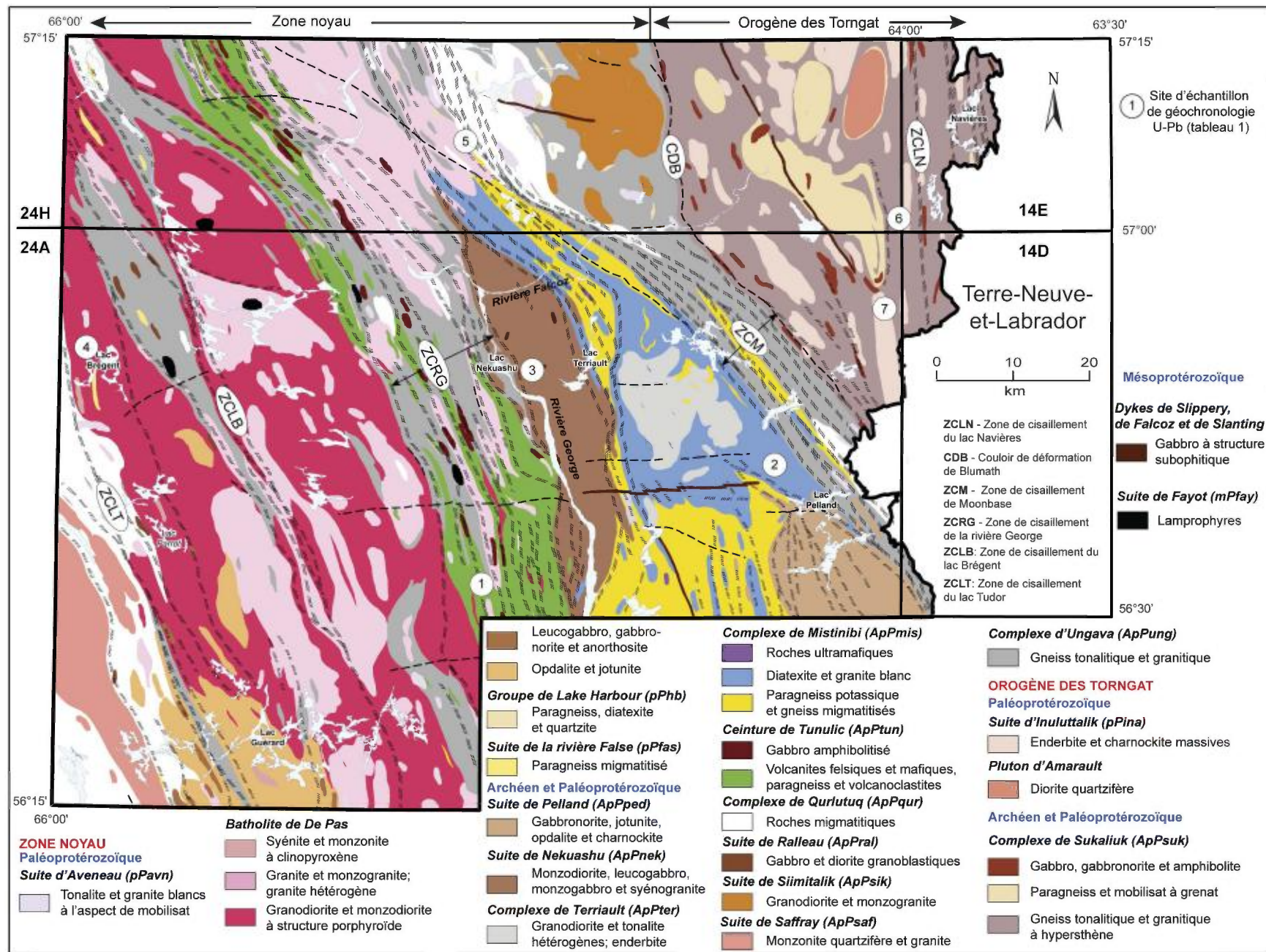
FIGURE 4 - Géologie simplifiée de la région du lac Brisson.
