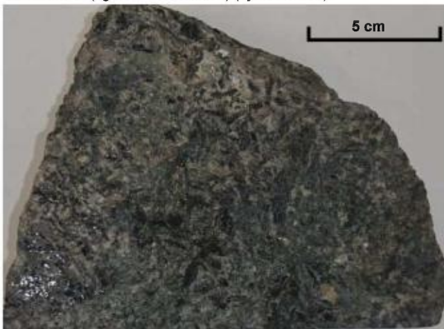
PHOTO 21 - Lamprophyre mélanocrate massif de la Suite de Fayot (mPfay). Échantillon riche en biotite et minéralisé en éléments des terres rares (site 1, figure 14 et tableau 2).
