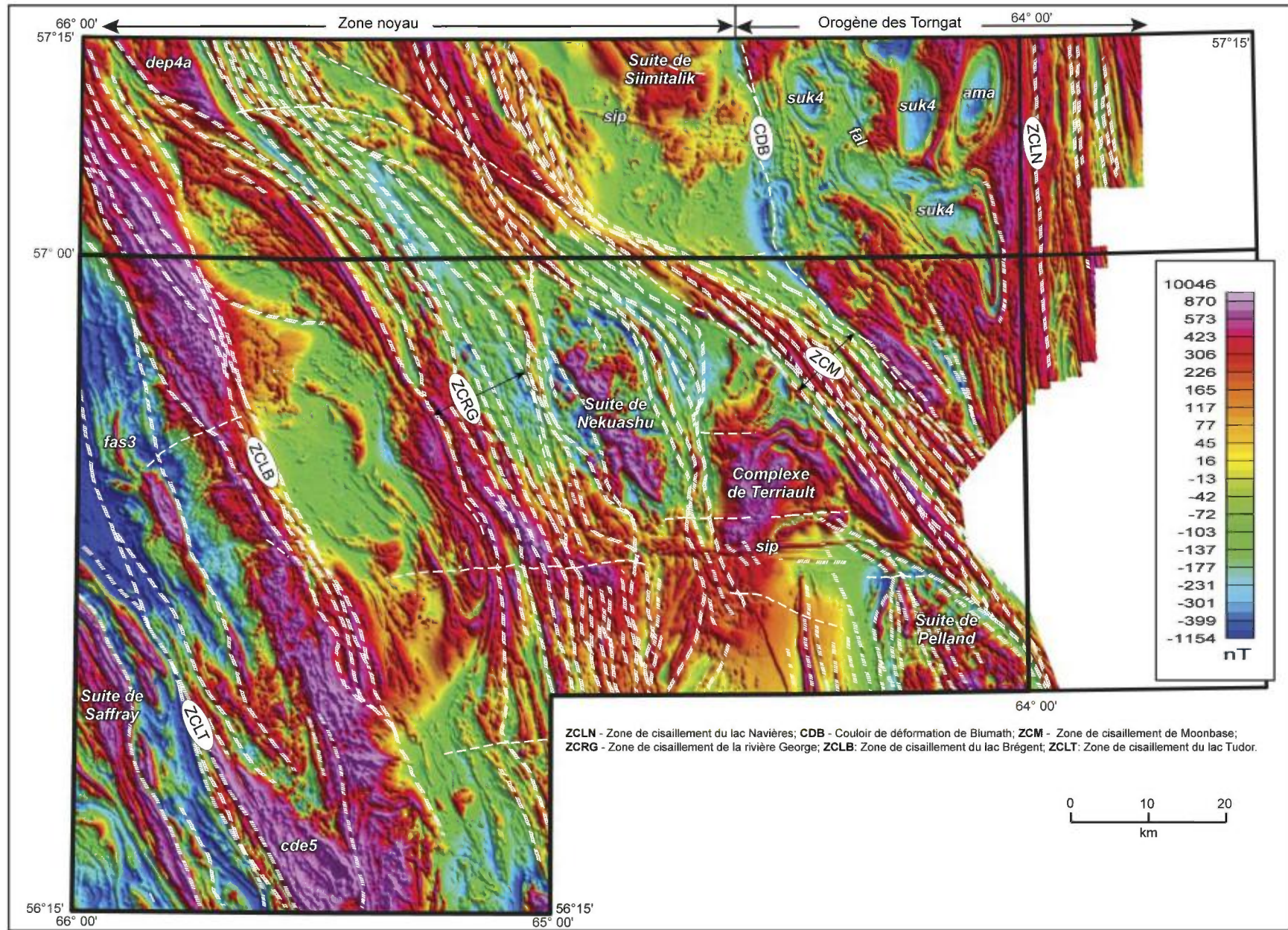
FIGURE 5 - Composante résiduelle du champ magnétique total de la région du lac Brisson.
