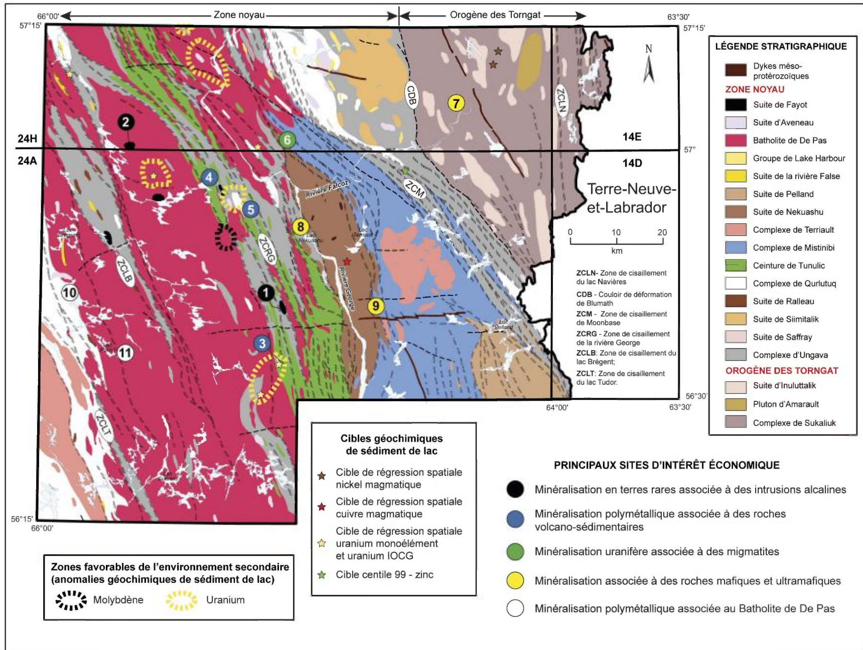
FIGURE 12 - Localisation des principaux sites d'intérêt économique de la région du lac Brisson. Les numéros font référence aux sites décrits au tableau 2.
