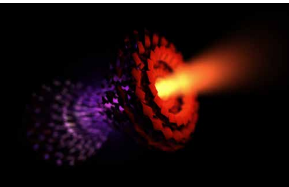
L'auteur aime ce dessin d'artiste car il y voit un vaisseau spatial qui se déplacerait à des vitesses proches de celle de la lumière. À cette vitesse, le vaisseau se transforme sous les effets de la relativité. Crédit : Victor Glindås ( http://victorglindas.com )
