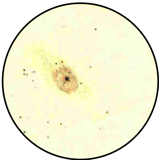
Dessin réalisé par l'auteur le 13 septembre 1982 avec un télescope de 310 mm (12") f/15 et un oculaire de 60 mm (G = 77,5×).
