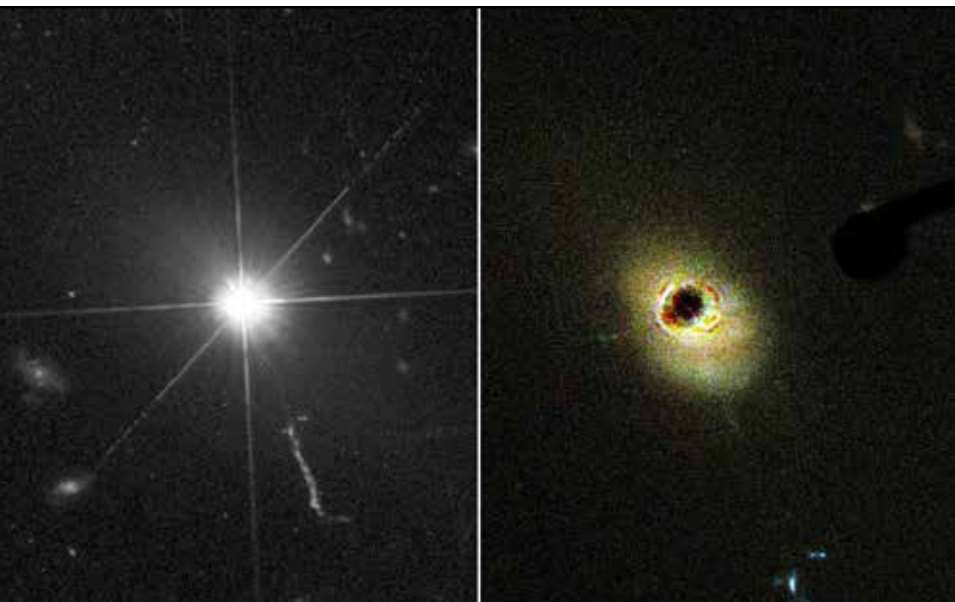
À gauche : Le quasar 3C 273, avec une magnitude apparente de 12,9, est le seul quasar observable avec un équipement d'amateur. Il est situé à 1,9 milliard d'années-lumière de la Terre, dans la constellation de la Vierge. Sa magnitude absolue est de -26,7 , cela veut dire que s'il était à une distance de 33 années-lumière, cet objet brillerait dans le ciel aussi fortement que le Soleil. Crédit : NASA et J. Bahcall (IAS).
