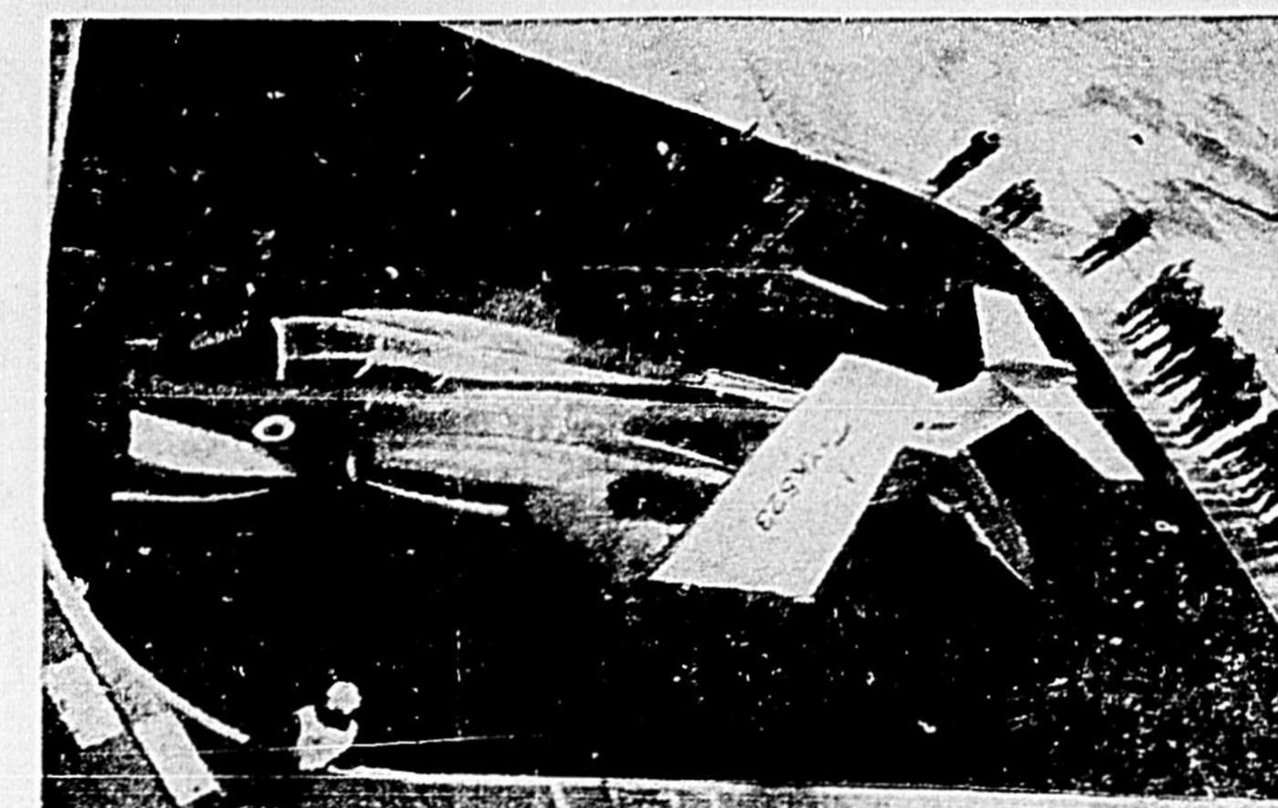
Le dernier en date des bombardiers atomiques de la Grande-Bretagne, le N.A. 39 (Blackburn), vient de faire avec succès ses essais de décollage et d'appontage sur le porte-avions VICTORIOUS. C'est un appareil d'attaque capable de voler très bas. On voit sur notre cliché le N.A. 39 ailes et nez repliés et freins pneumatiques (à l'arrière du fuselage) largement ouverts; on est en train de le faire descendre dans son hangar sous le pont principal du porte-avions, ses essais terminés. Au cours de ces derniers, le N.A. 39 a fait plus de trente décollages et appontages en trois jours et demi. Lance par la catapulte à vapeur du porte-avions, cet avion très complexe reprend contact avec le sol à une vitesse très réduite, ainsi qu'on a pu le constater. Le N.A. 39, dont les premiers essais de vol ont eu lieu il y a 21 mois, peut transporter des bombes classiques ou nucléaires. Il vole à une vitesse voisine de celle du son et à une hauteur lui permettant de passer sous la couverture radar de l'ennemi. Cet appareil, qui sera en service dans l'Aéronautique Navale de la Marine de Guerre avant la fin de l'année, est propulsé par deux turbo-reacteurs "Gyron Junior" (de Havilland).
