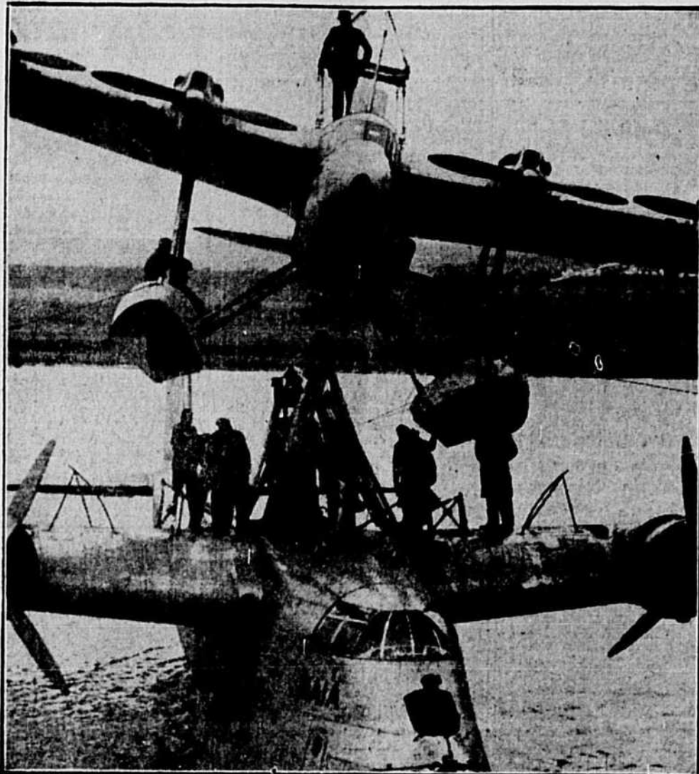
Le hydravion anglais "Mercury", attendu ce matin à Boucherville, terme d'une audacieuse envolée transatlantique entreprise, hier, depuis Foynes, Eire, n'est que la moitié d'un appareil volant, invention du major Robert Mayo et dont on voit, sur cette photo, les deux parties distinctes. Hier, le départ fut conjoint, au-dessus de Foynes, mais une fois au large des côtes de l'Eire, le "Maia" a catapulté le "Mercury" qui a continué seul le voyage.
