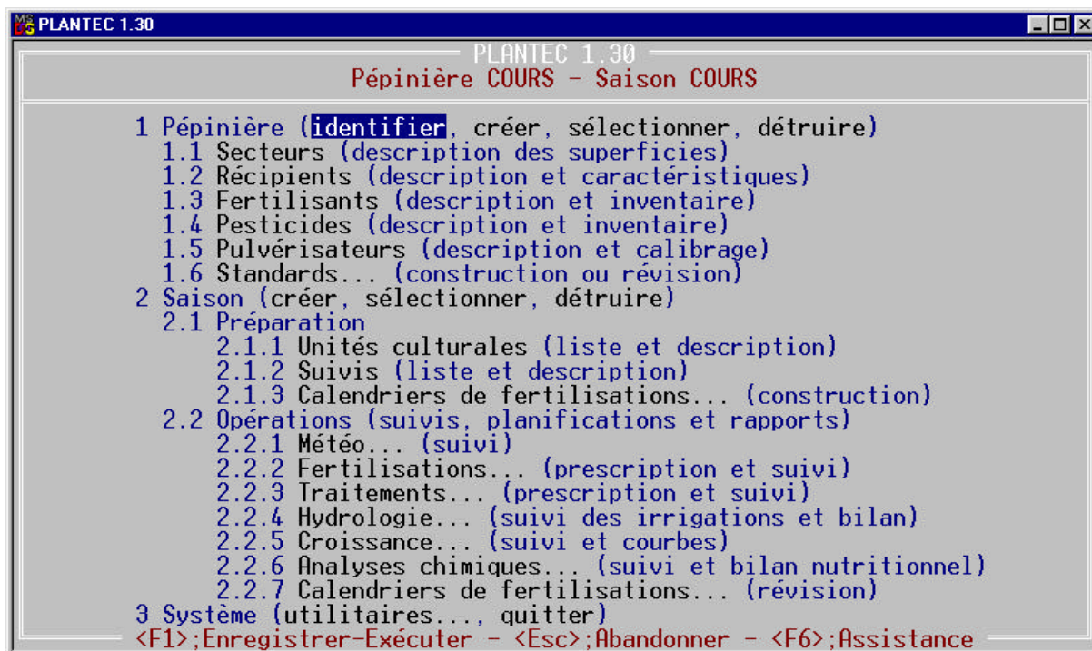
Figure 2. Écran principal de PLANTEC.
