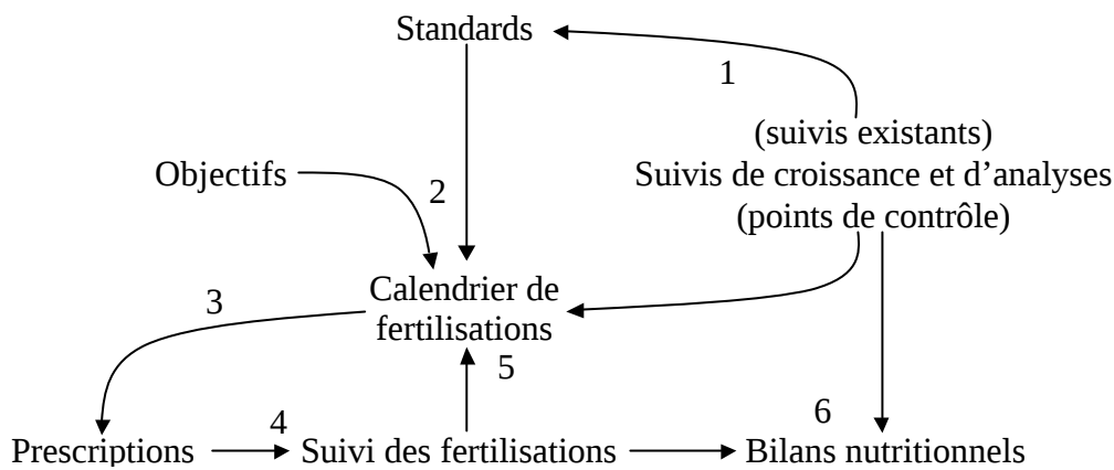
Figure 1. Le fonctionnement de PLANTEC : des suivis existants sont utilisés pour établir les standards (1). Les standards sont ajustés en fonction des objectifs de croissance pour construire des calendriers de fertilisations (2). Les calendriers alimentent une fonction qui guide la préparation et l'application des solutions fertilisantes (3). Les fertilisations réalisées sont mémorisées (4). Les suivis (points de contrôles) et les fertilisations mémorisées servent à la révision périodique des calendriers (5) et au calcul des bilans nutritionnels (6).
