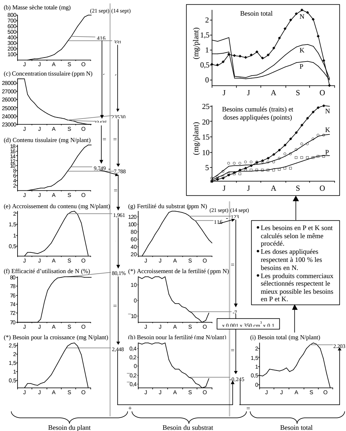
Figure 3. Calculs pour la fertilisation du 14 septembre qui donnent une vue d'ensemble de la progression saisonnière des paramètres. Les lettres qui identifient les graphiques correspondent à celles des colonnes du calendrier de fertilisations du tableau 1. Les graphiques marqués d'un astérisque (*) proviennent d'un calcul intermédiaire qui n'apparaît pas dans le calendrier. Les graphiques illustrés sont de même forme que ceux produits par PLANTEC.
