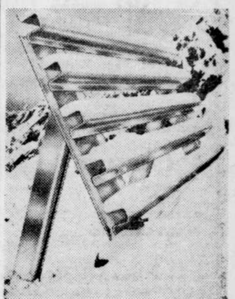
Le paraneige robuste mais léger en alliage 57S trois-quarts dur ne s'altère pas et il peut supporter une charge de 12,5 tonnes au mètre. Le matériau a été fourni par Aluminiumwerke A. G. Rorschach.
