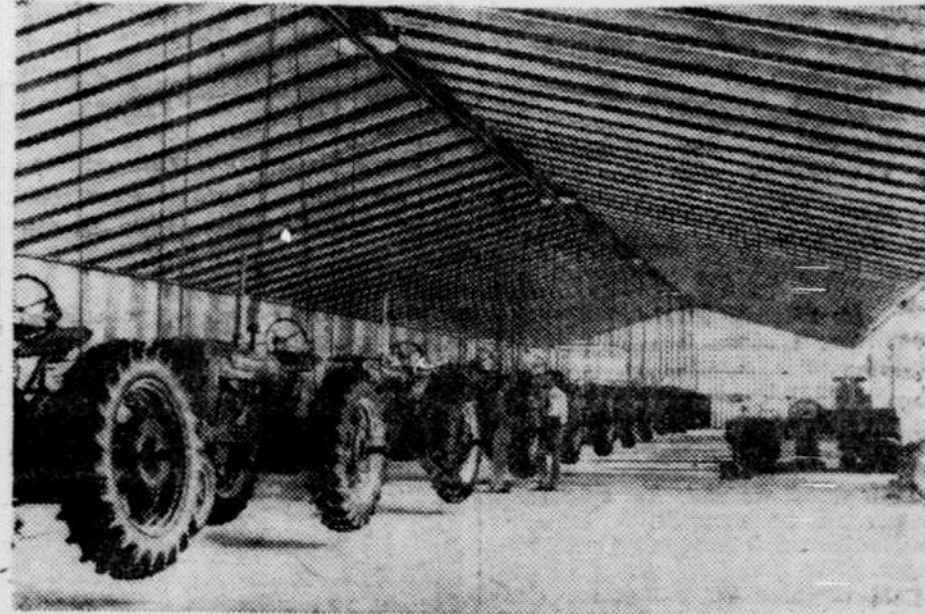
On jugera de la robustesse des bâtiments Behlen sans charpente par cette photographie où l'on voit 14 tracteurs d'un poids total de 32 tonnes suspendus au toit.
