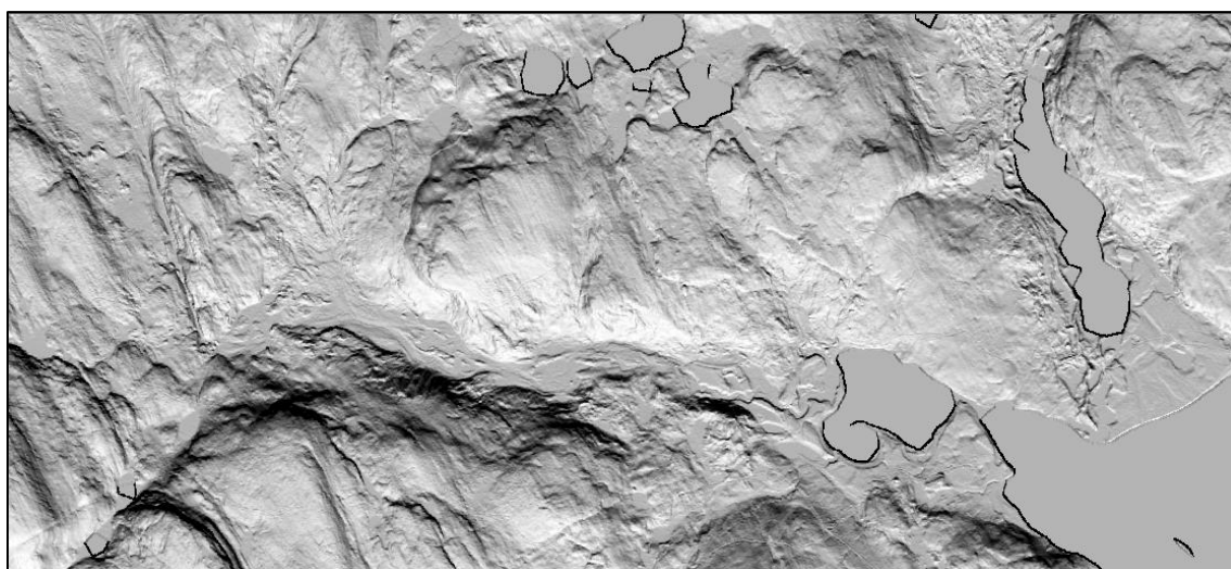
Exemple 3 : MNT_ombré à 180° d'azimut (sud) dont la topographie est inversée.
