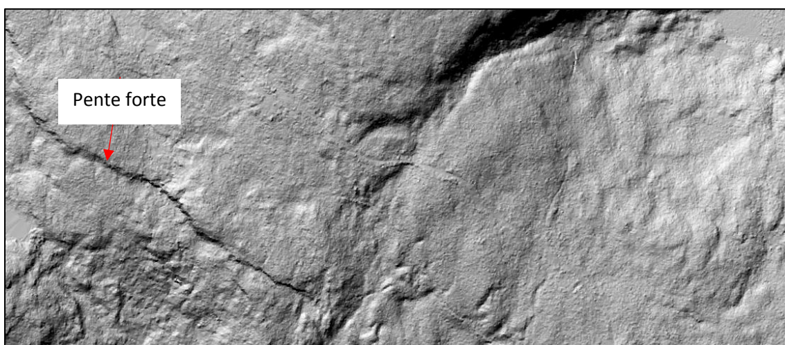
Exemple 2 : MNT_ombré à 320° d'azimut et un facteur Z de 2.
