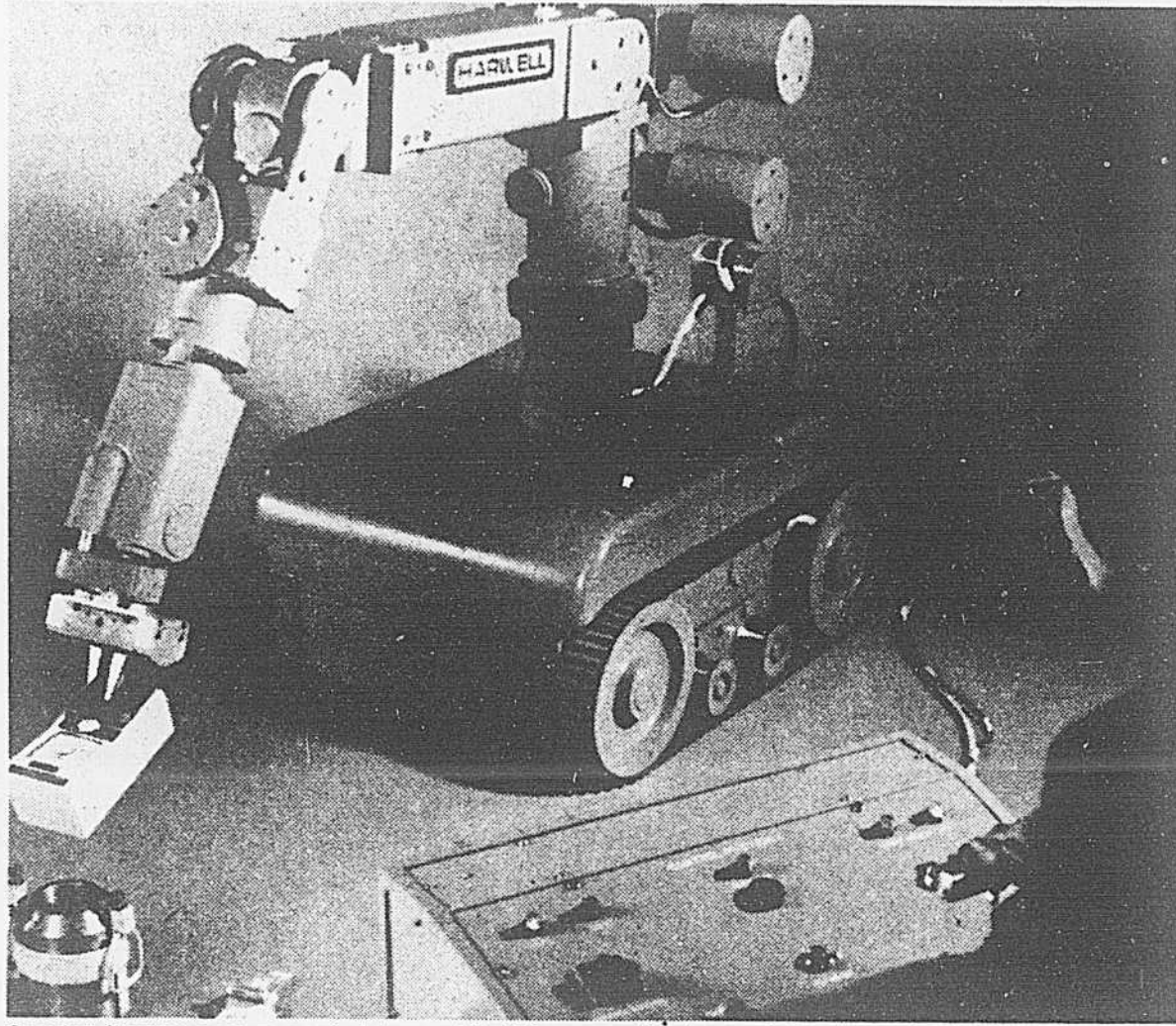
Ce robot électrique est un manipulateur mobile télécommandé, mis au point par la division de mécanique de Harwell pour le laboratoire de développement des réacteurs nucléaires à Windscale, en Grande-Bretagne. Sur télécommande, il peut manoeuvrer dans des espaces restreints et soulever des charges de 36 kilogrammes. Ses chenilles lui permettent de franchir des obstacles de dix centimètres et des pentes de 15 degrés. Il peut se déplacer à la vitesse d'un mètre/seconde.
