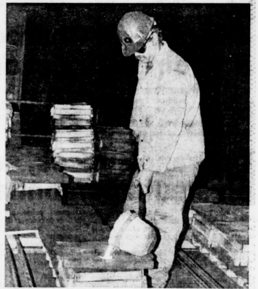
La fonte en fusion est coulée dans le moule en sable synthétique, où elle durcira en cinq minutes.
