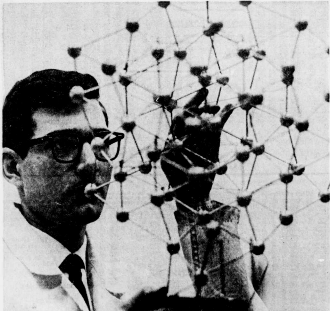
Au Centre de recherches Noranda, à Pointe-Claire, un chercheur devant la structure cristallographique du sélénium. Chaque petite sphère correspond ici à un atome de métal; les bâtonnets qui les unissent représentent les distances et les liaisons interatomiques. Le sélénium a des applications comme matériau semi-conducteur, en Xéographie notamment, et dans les redresseurs de courant.
