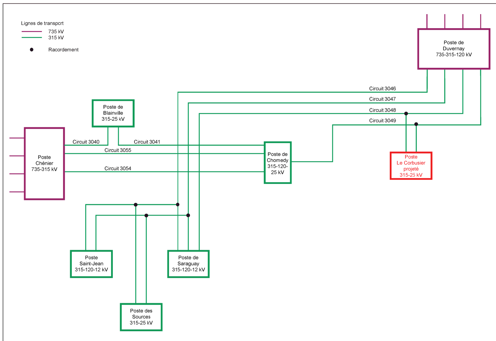
Figure 2-2 : Schéma unifilaire du réseau à haute tension – Situation future
