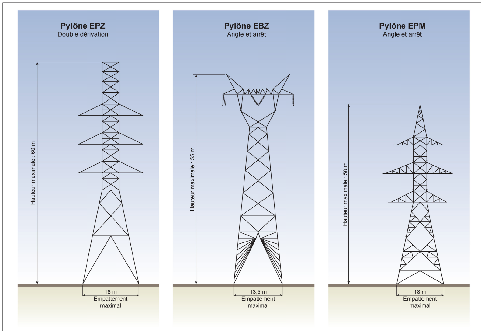
Figure 2-3 : Supports types de la ligne de raccordement à 315 kV projetée
