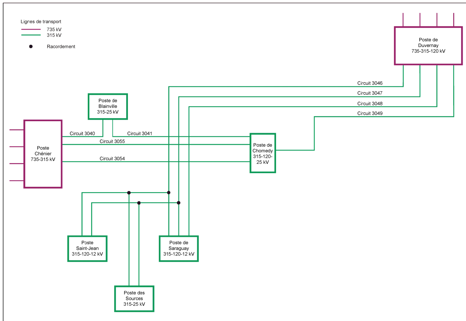
Figure 2-1 : Schéma unifilaire du réseau à haute tension – Situation actuelle
