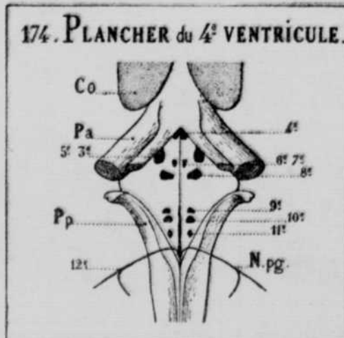
174. — PLANCHER DU 4e VENTRICULE.
