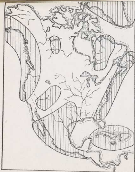
Le « continent américain » à l'époque ordovicienne — 400.000.000
