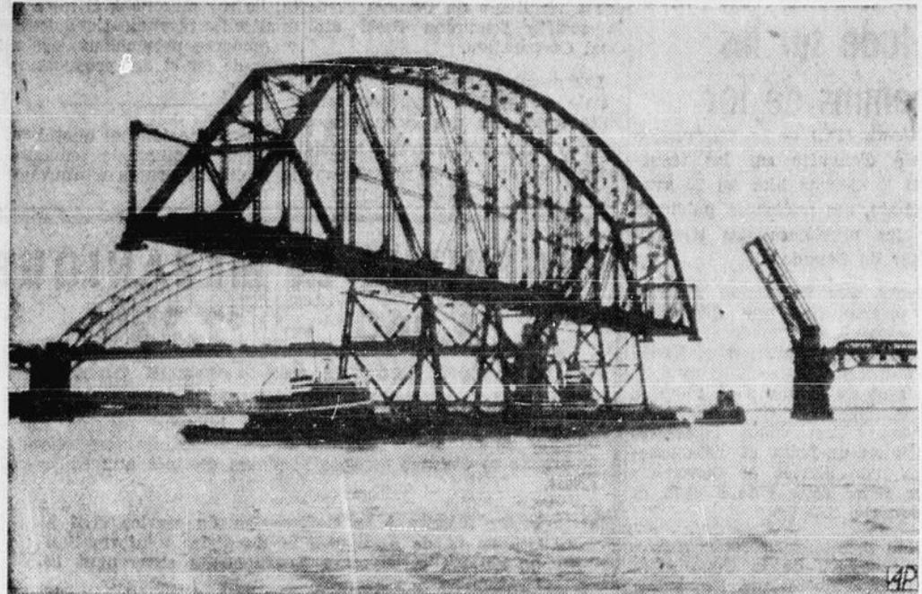
QUAND DEUX PONTS SE RENCONTRE...
