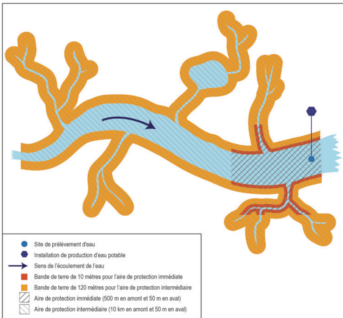
Figure 8 : Aires de protection immédiate et intermédiaire d'un site de prélèvement situé dans une rivière
