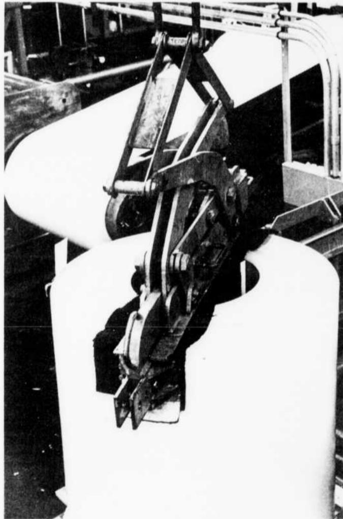
DES ROULEAUX DE TOLE d'aluminium prépeinte, tels que fabriqués à l'une des deux chaînes de peinture de l'usine Alcan de Kingston, répondent aux besoins croissants du marché, surtout dans le domaine de la construction de bâtiments et le transport. L'Alcan a fait part de son intention d'agrandir ses installations de pré-peinture au cours de 1969 afin de mieux servir ce marché en plein essor. (Autres détails à la page 12).
