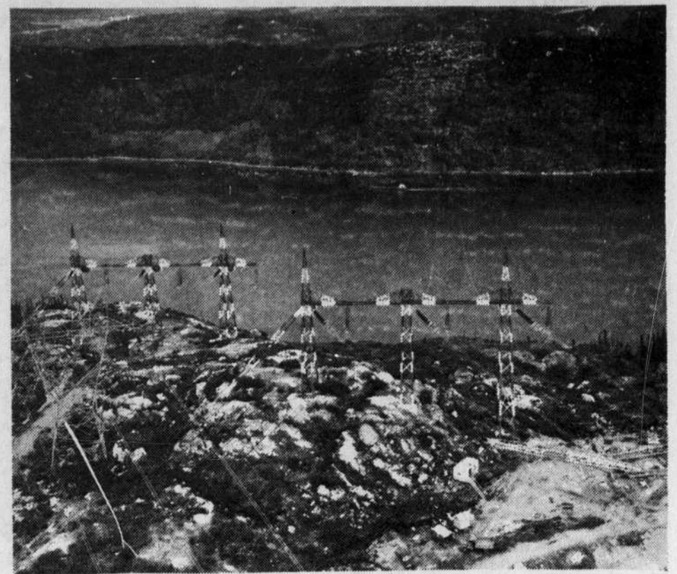
Ligne de transmission de 735.000 volts venant de Manicouagan à l'approche du Saguenay.
