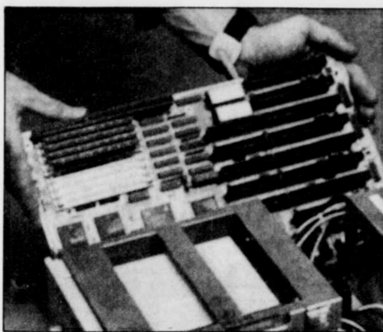
Sur cette photo, on aperçoit (à droite, sous la main), les connecteurs d'extension de cet appareil: deux 8-bit (les plus petits, en haut) et cinq connecteurs 16-bit.
