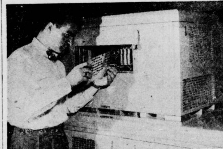
ON VOIT CI-DESSUS le centre d'entretien du nouvel outillage de commutation à barres transversales A-A de Montréal. Advenant une défectuosité, celle-ci est automatiquement rapportée aux instruments de vérification, et des techniciens de la compagnie Bell peuvent immédiatement la rectifier.
