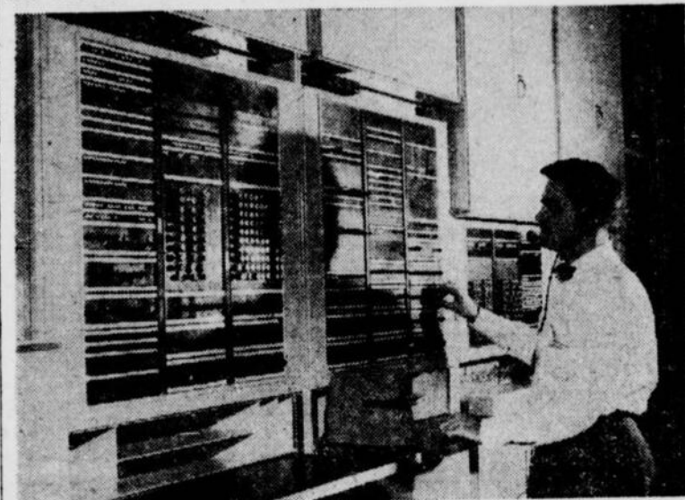
ON VOIT CI-DESSUS le centre d'entretien du nouvel outillage de commutation à barres transversales A-A de Montréal. Advenant une défectuosité, celle-ci est automatiquement rapportée aux instruments de vérification, et des techniciens de la compagnie Bell peuvent immédiatement la rectifier.
