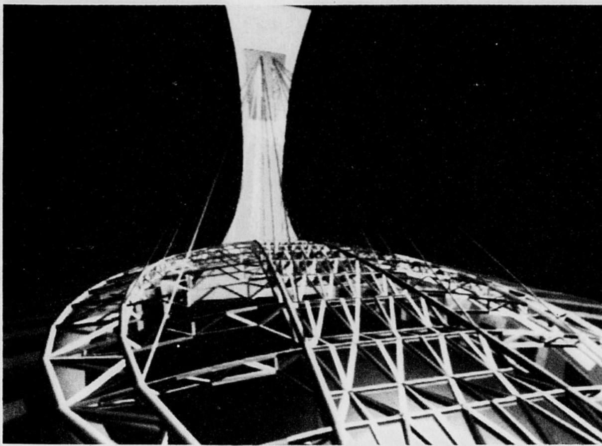
La RIO a présenté cette maquette de son projet de toit fixe pour le Stade olympique. Les poutrelles seraient recouvertes de feuilles d'acier.
