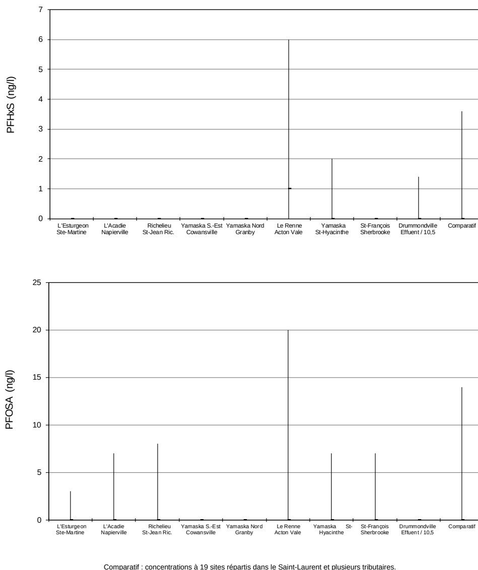
Figure 7 Sulfonate de perfluorohexane (PFHxS) et perfluorooctane sulfonamide (PFOSA) : concentrations maximum, minimum et médiane à chaque site d'échantillonnage
