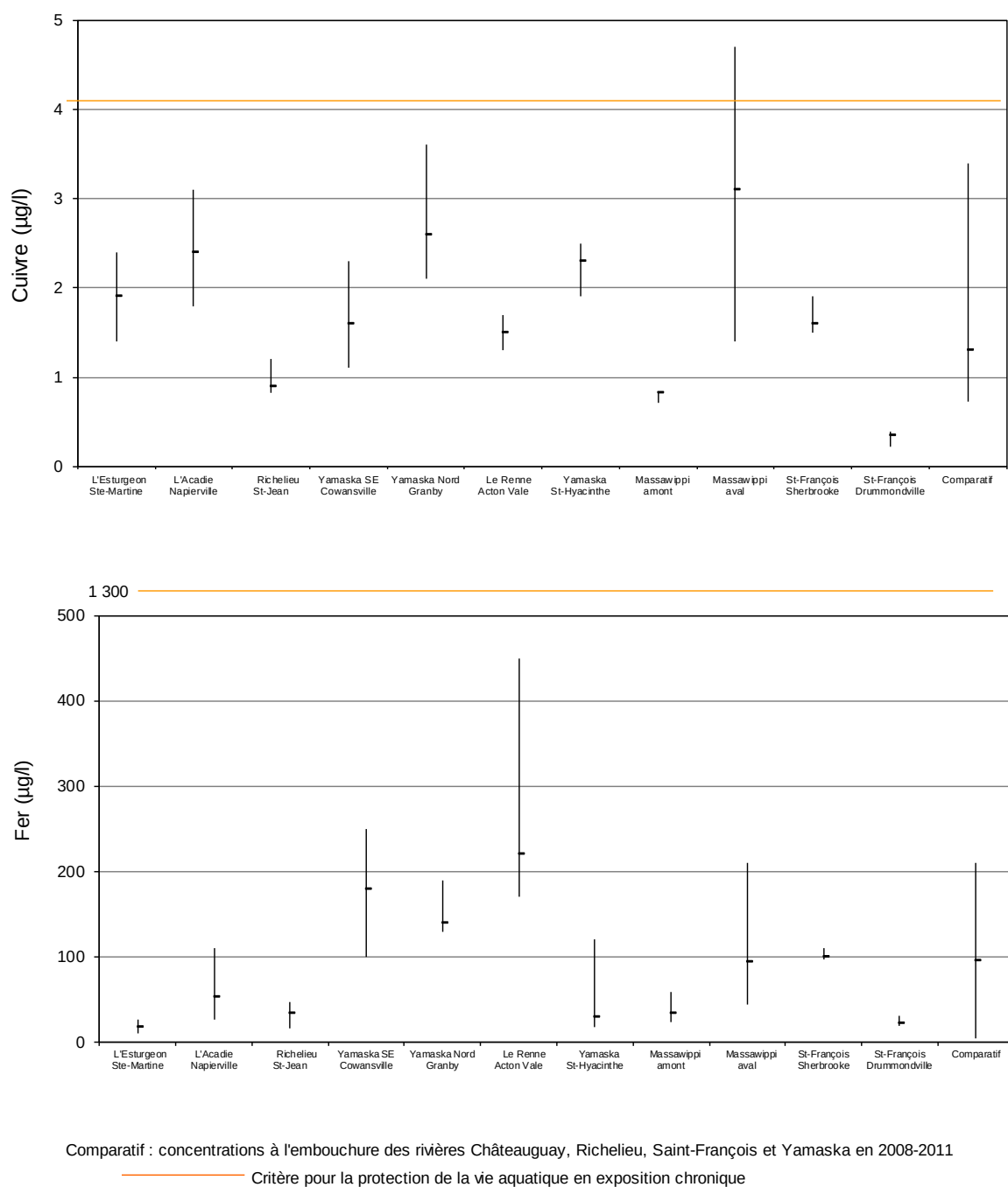
Figure 16 Cuivre et fer dissous : concentrations maximum, minimum et médiane à chaque site d'échantillonnage
