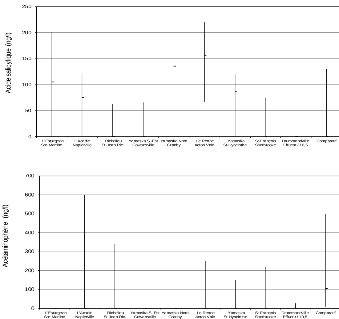
Figure 2 Acide salicylique et acétaminophène : concentration maximum, minimum et médiane à chaque site d'échantillonnage
