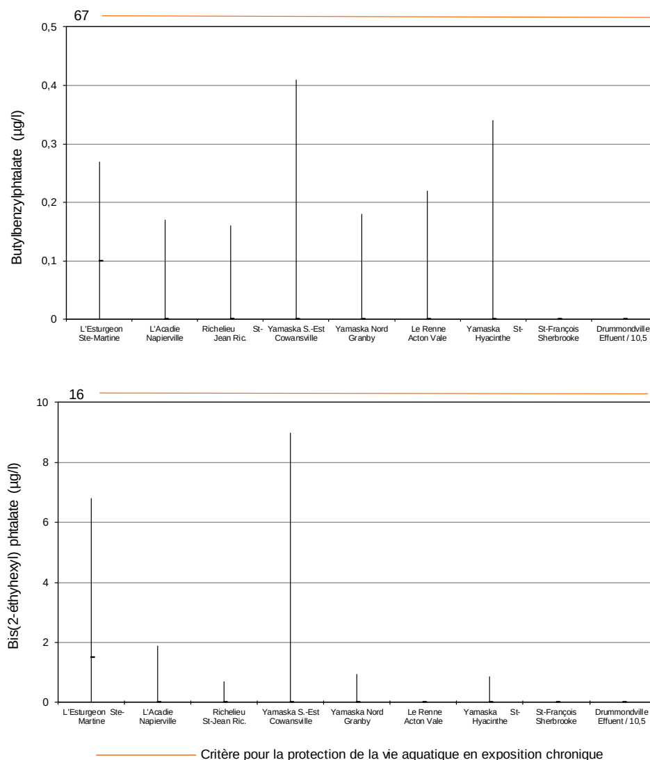
Figure 9 Butylbenzylphthalate et bis(2-éthylhexyl) phthalate : concentrations maximum, minimum et médiane à chaque site d'échantillonnage
