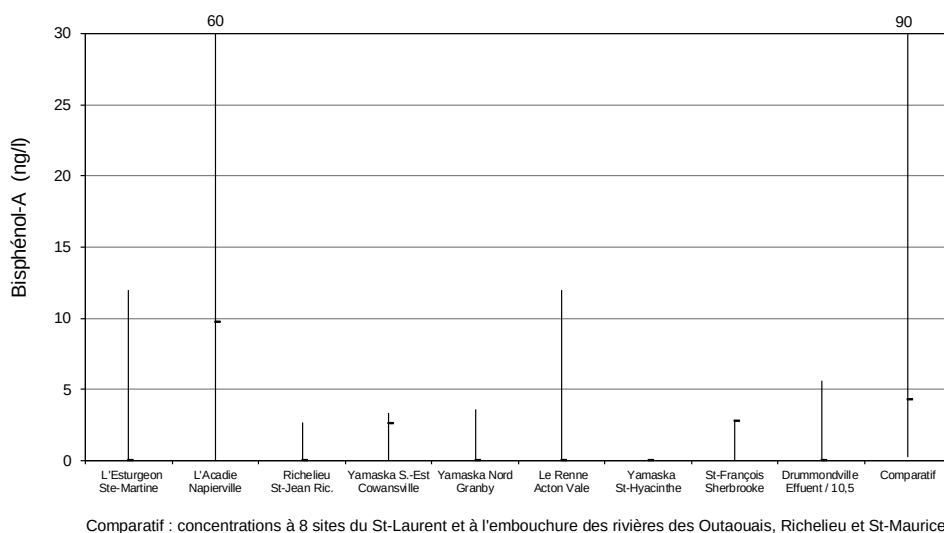
Figure 8 Bisphénol-A : concentrations maximum, minimum et médiane à chaque site d'échantillonnage
