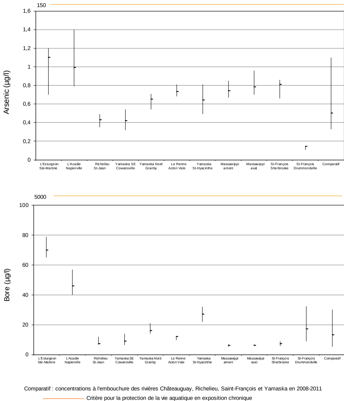
Figure 13 Arsenic et bore dissous : concentrations maximum, minimum et médiane à chaque site d'échantillonnage
