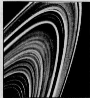
Les anneaux de Saturne vus par la sonde Voyager.
