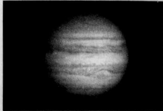
La photo de Saturne a été captée par la sonde Voyager, tandis que celle de Jupiter a été saisie par la sonde Cassini.
