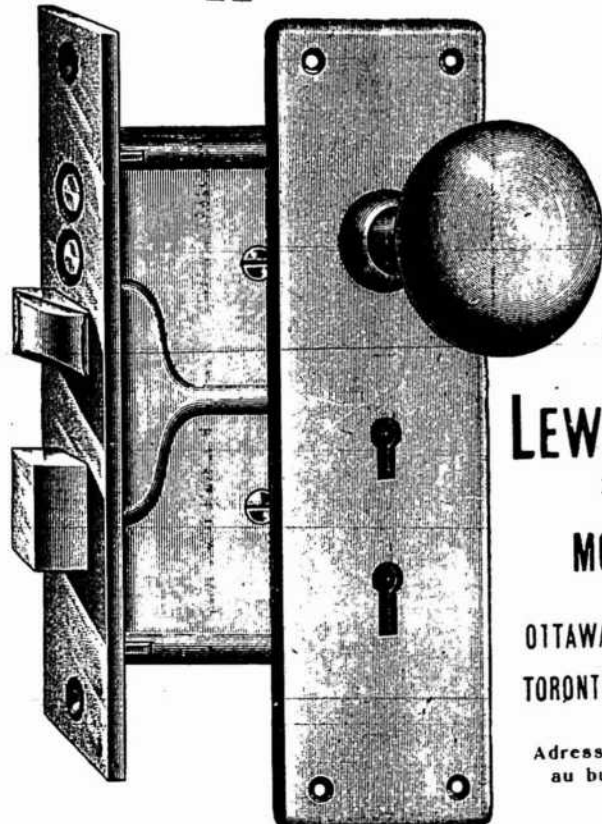
Garniture O. 2299. Pour Porte de Façade.
