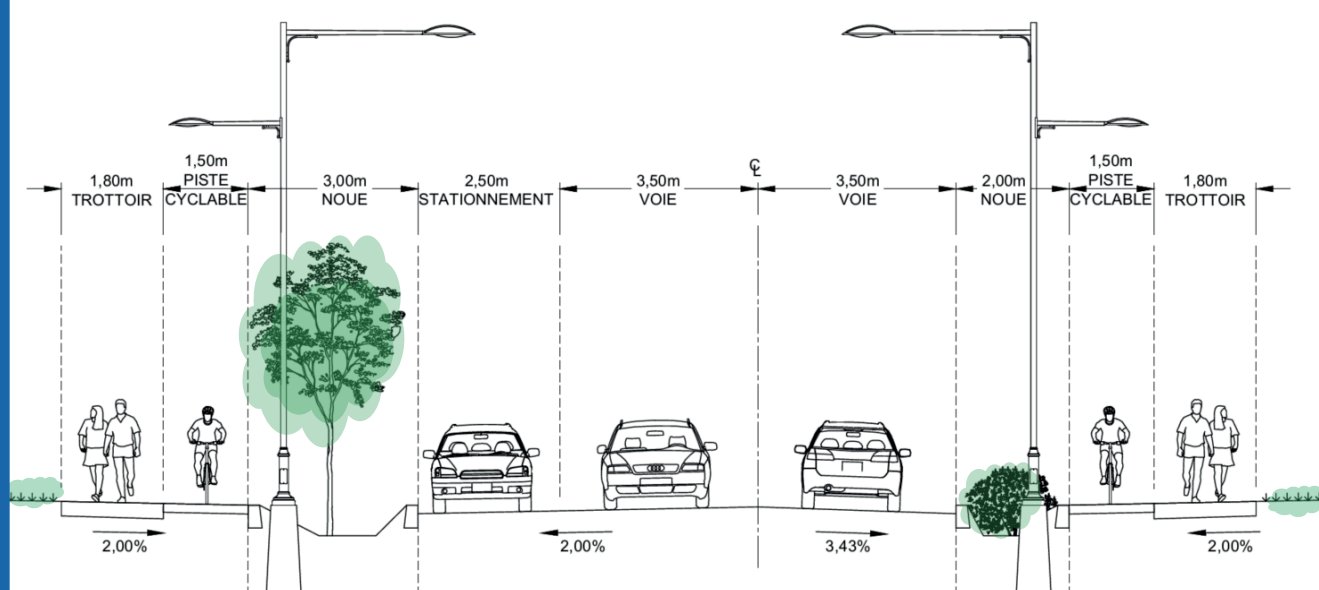
Coupe de la route De Lotbinière après les travaux
