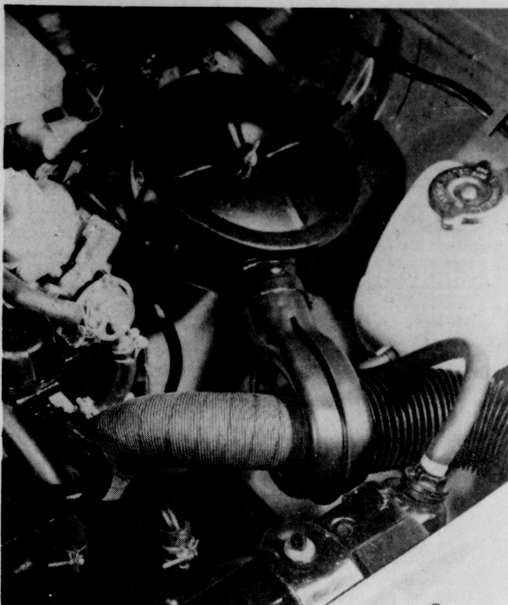
Le dispositif de contrôle de température et d'air installé sur la Marina destiné à l'exportation. Le boyau (à gauche) tire l'air chaud qui circule autour du collecteur d'échappement. Le boyau de droite reçoit l'air froid et les deux courants d'air se mélangent automatiquement pour former une température constante.
