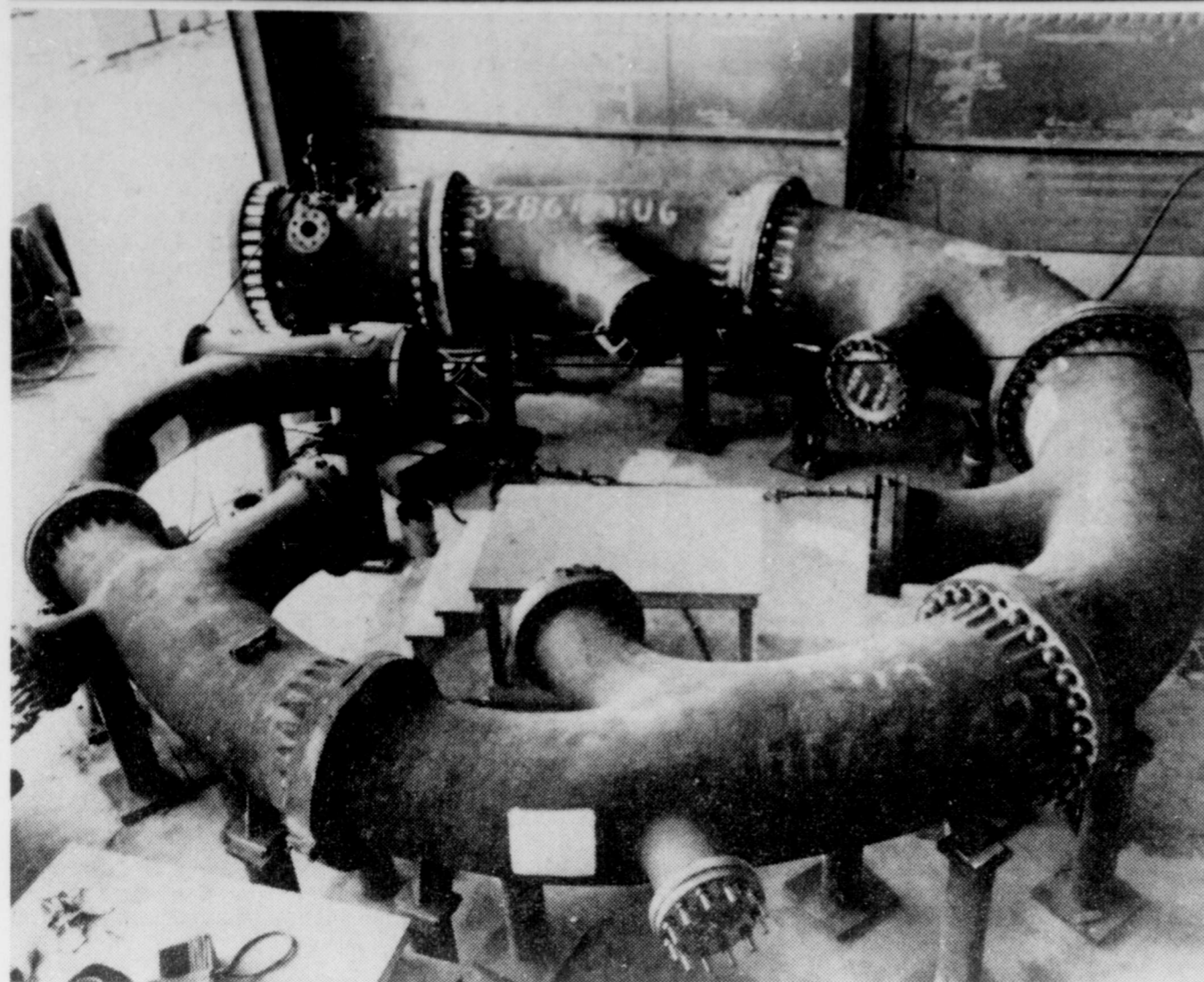
Une des sections des turbines et alternateurs en voie de construction par Marine industrie limitée dans ses usines à Tracy, pour INECEL (Instituto Ecuatoriano de Electrificación) et qui sont destinées au projet de Pisayambo en Equateur, Amérique du Sud.
