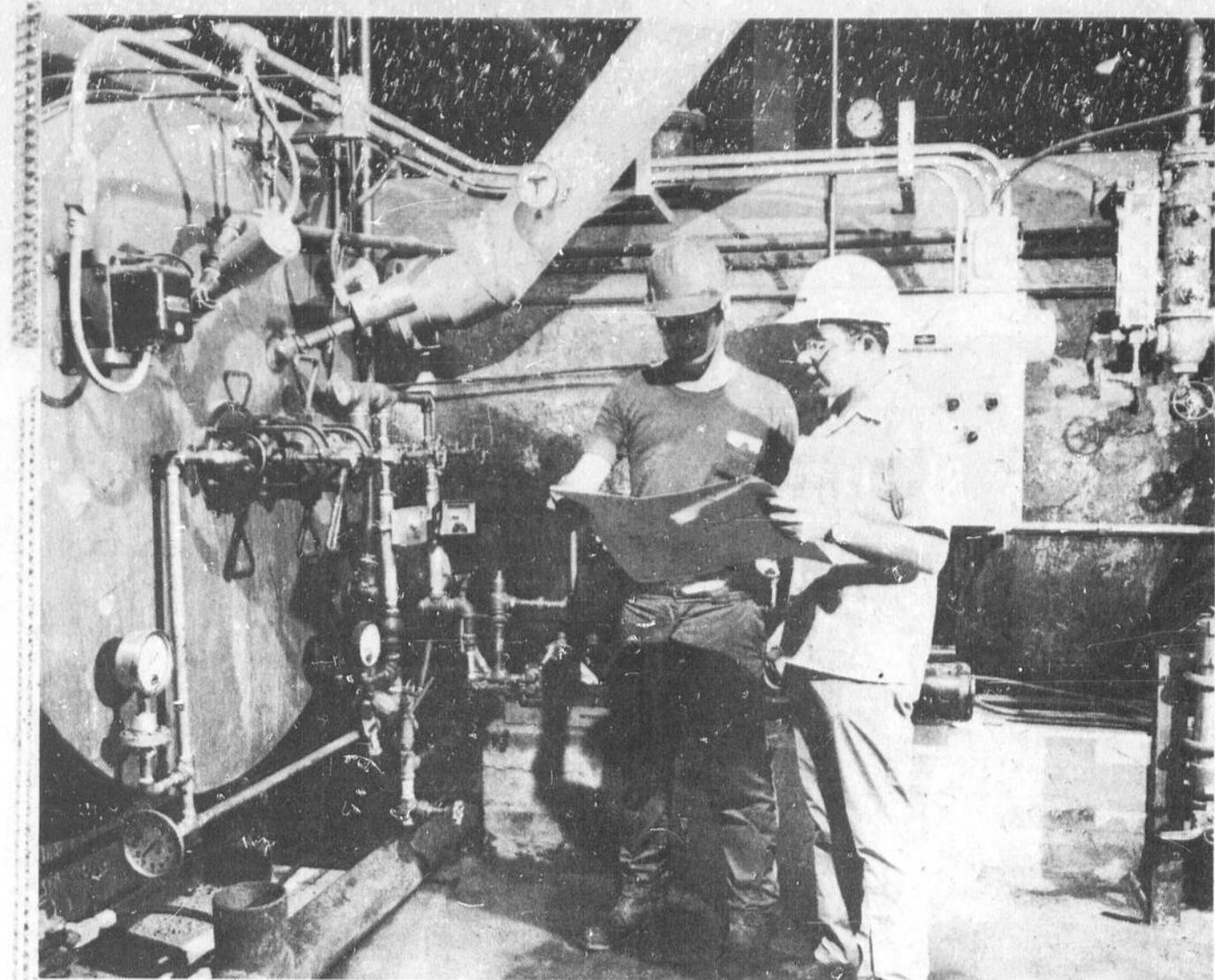
EDDY LUTTE CONTRE LA POLLUTION — On voit ici une partie de l'outillage destiné à récupérer l'anhydride sulfureux et réduire ainsi la pollution. Cette nouvelle usine pilote de récupération a été installée à l'usine de bisulfite de la compagnie E. B. Eddy. On aperçoit sur la photo M. Jacques Thériault, employé de la firme Eddy, discutant de l'efficacité pratiquée de l'outillage avec un ingénieur de la CIL.
