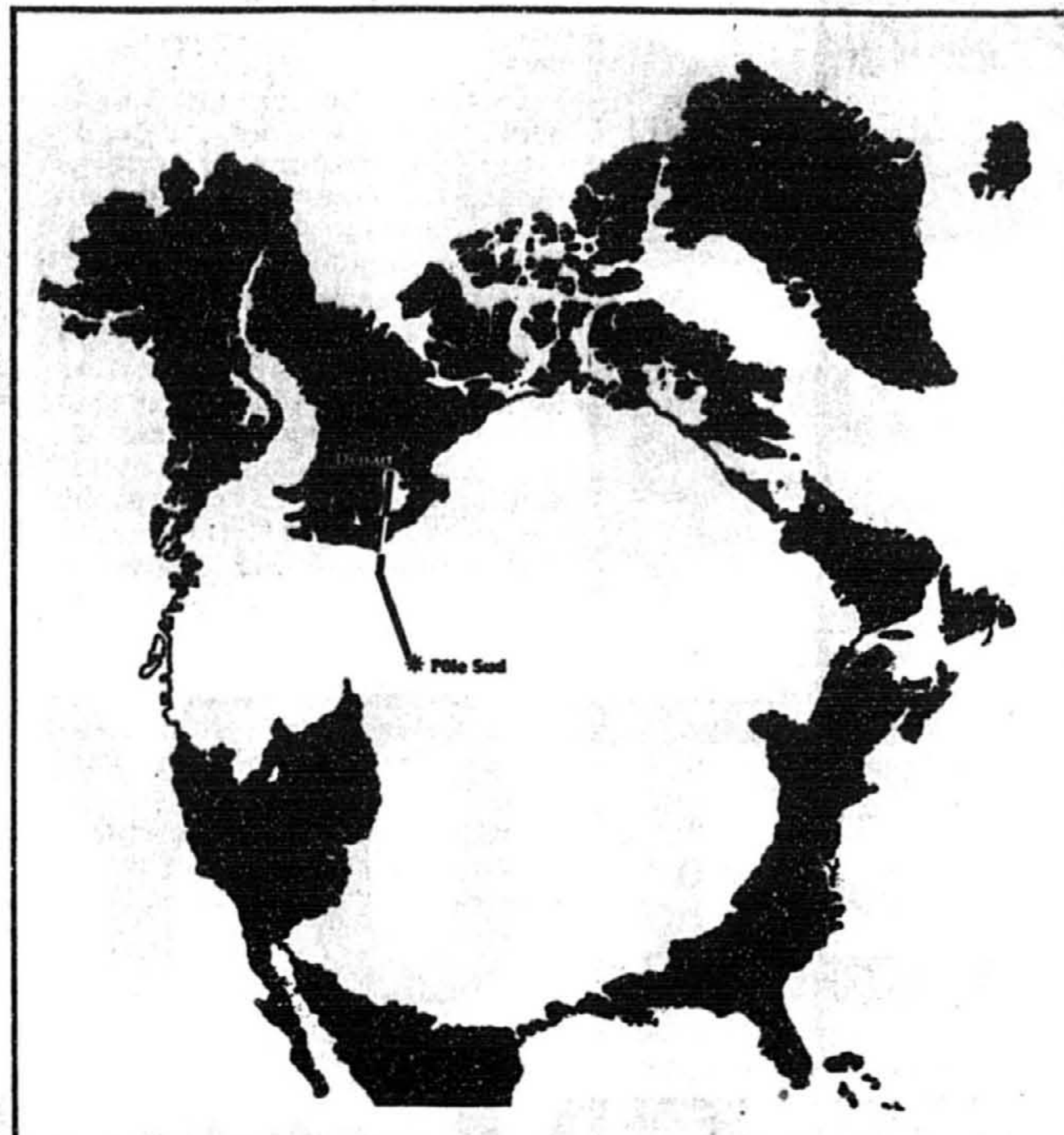
Le continent Arctique, 13 millions de km 2 recouvriraient la presque totalité de l'Amérique du Nord.
