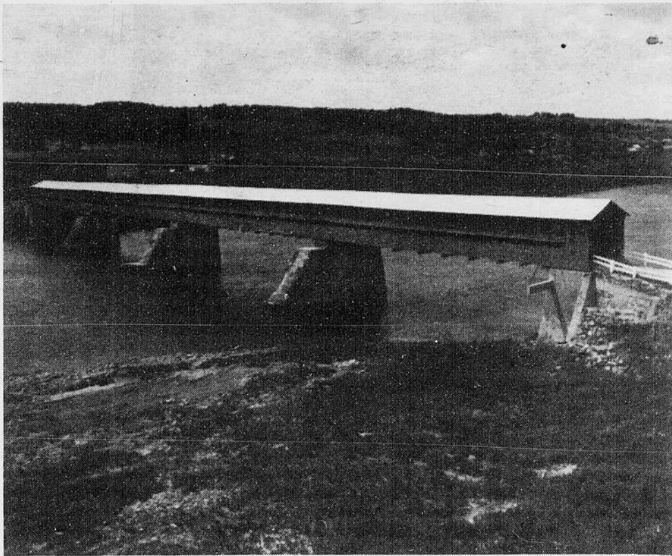
La rivière Chaudière dans la Beauce pourrait alimenter quatre centrales avec des potentiels respectifs de 3,5, .47, .25 et 1,55 mégawatts.
