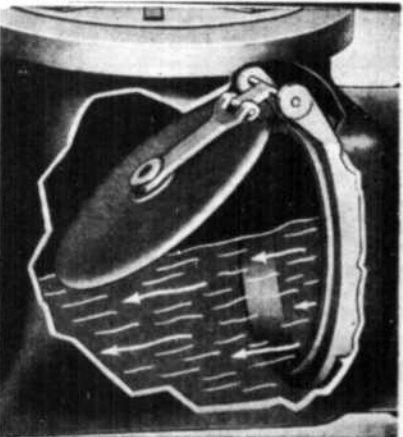
LES EAUX USEES de la maison passent par le clapet en faisant ouvrir le couvercle.
