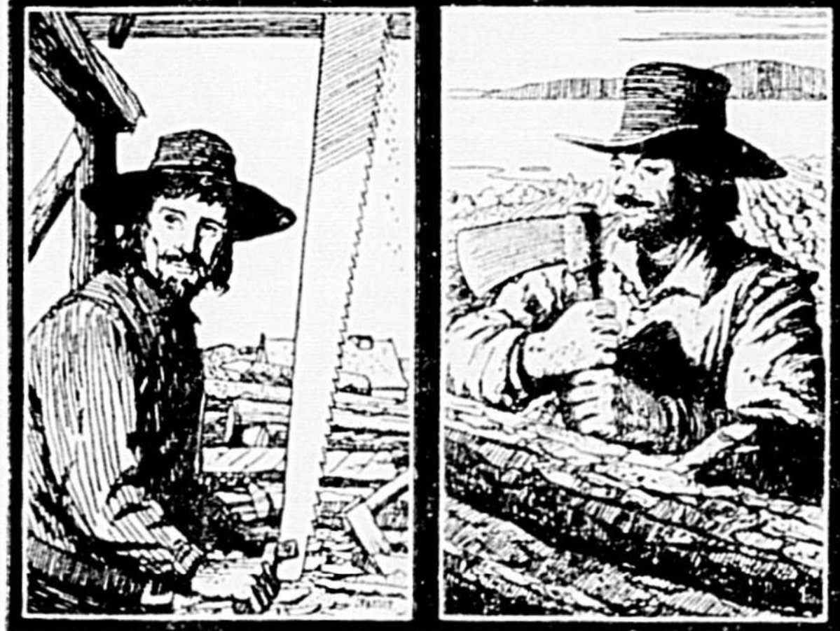
Pelletier-Peltier
