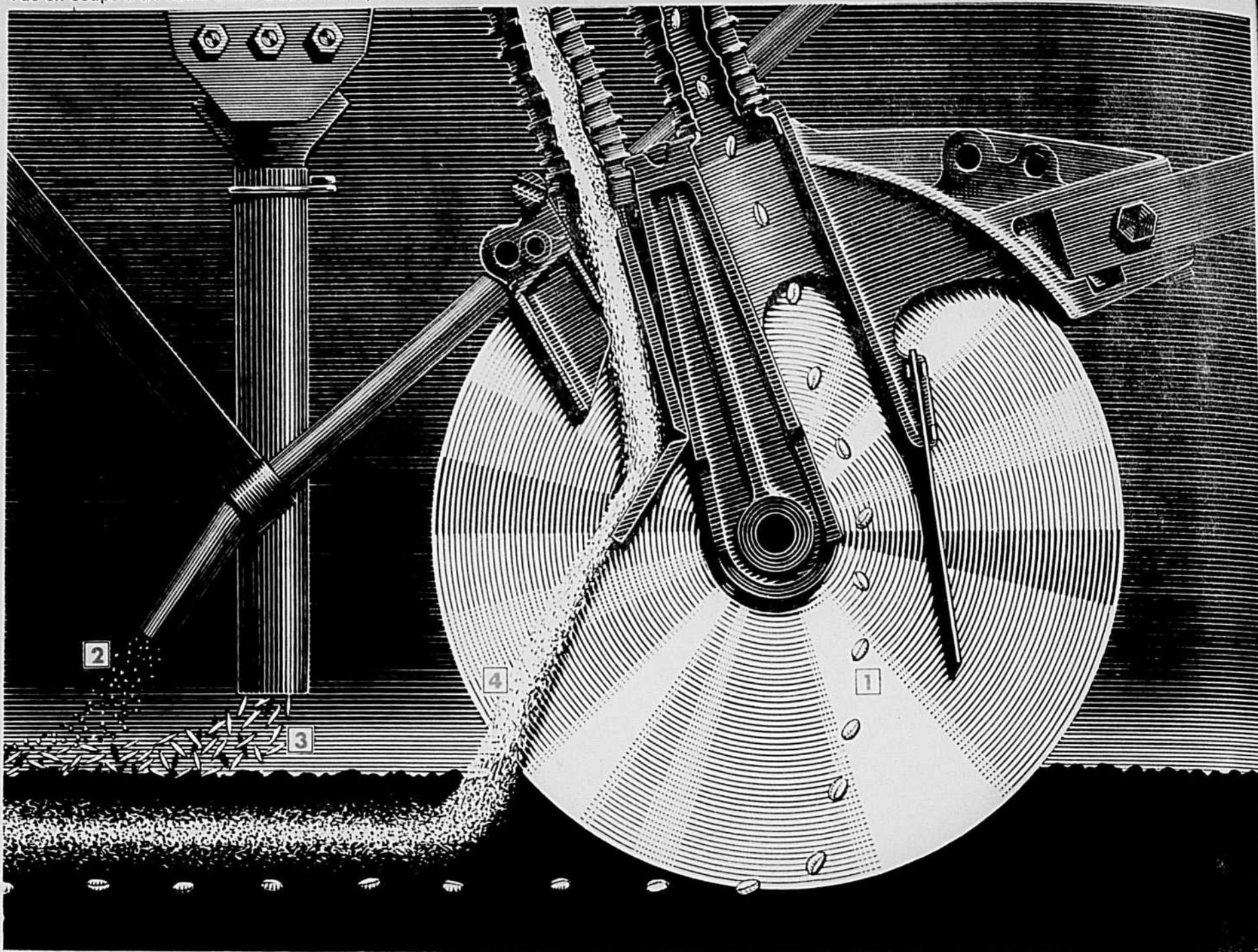
Distribution séparée (ou diverses combinaisons) des 1 céréales, 2 fines graines, 3 brome et 4 engrais.
