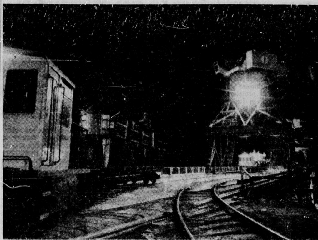
LE TRAVAIL SE CONTINUE LA NUIT — Même pendant la nuit les convois transportent le ciment à la digue principale de Mountain Chute de l'Hydro-Ontario sur la rivière Madawaska. Les convois voyagent 24 heures
