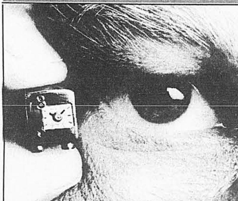
L'horloger suisse Fredy Suess nous montre la plus petite pendule mécanique du monde qui pèse 1,9 g. Elle a été construite à partir de 150 pièces et mesure 9,9 mm.
