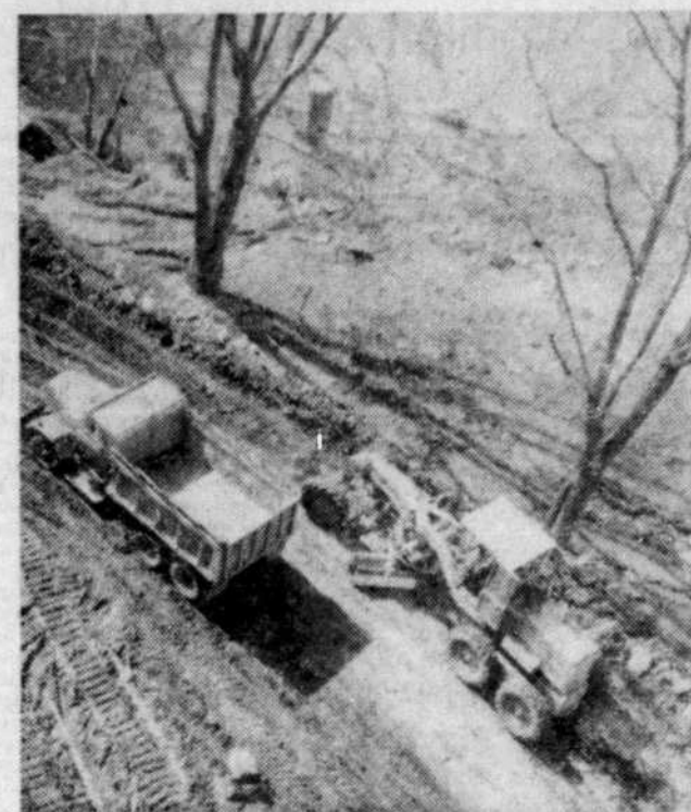
Dès qu'un camion est déchargé, la niveleuse entre en action...
