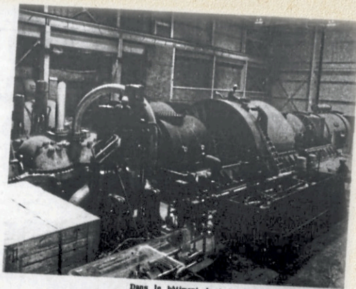
Dans le bâtiment du turbo-alternateur de la centrale nucléaire de Gentilly, les techniciens travaillent à la finition de la turbine située au centre et de l'alternateur au fond à droite.
